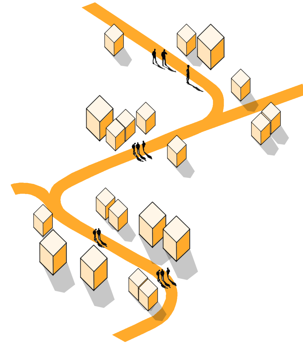
Phase n...
