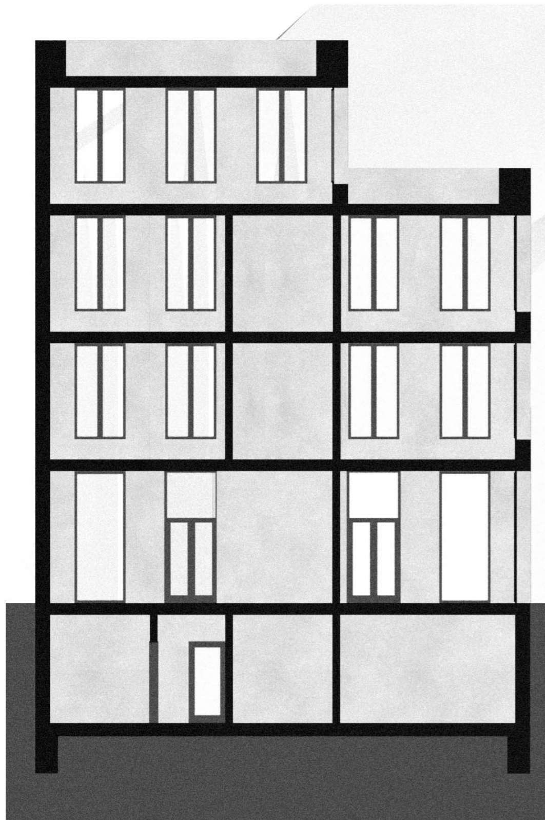
ŘEZ PŘÍČNÝ
