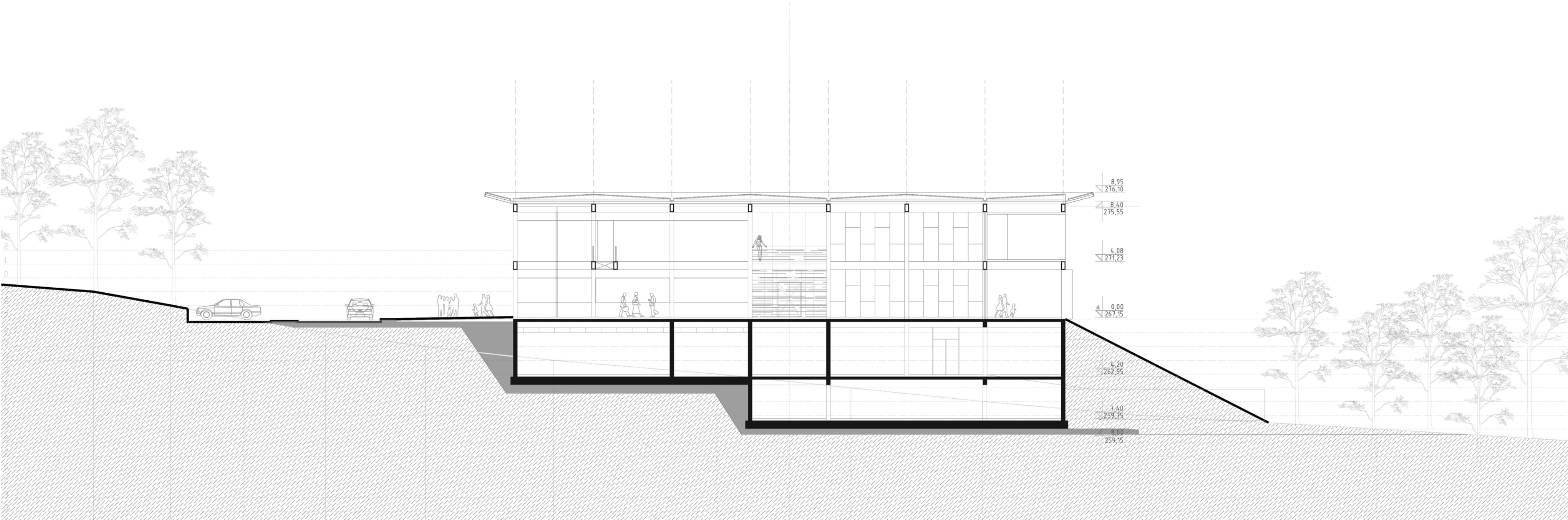
Section A-A 1:200
