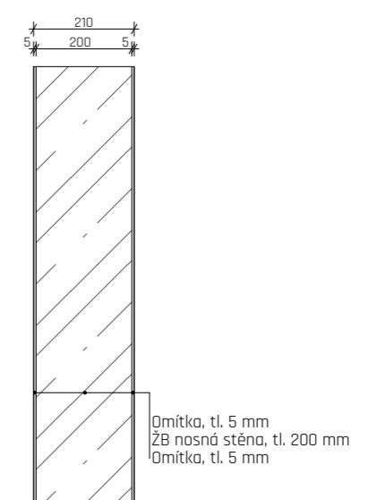
S5 VNITŘNÍ STĚNA ŽB 200
