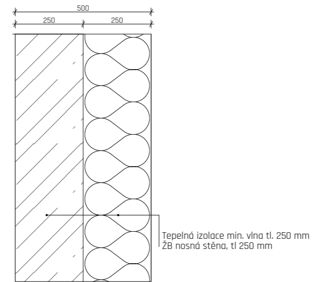
S3 OBVODOVÁ STĚNA U VELEJŠÍ BUDOVY
