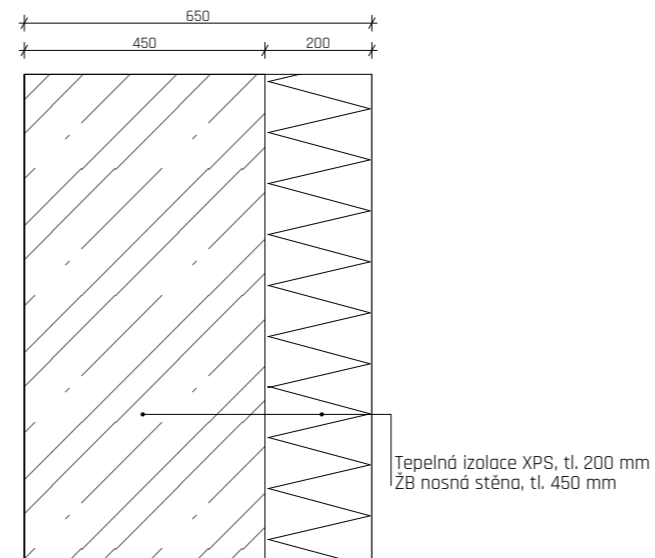
S8 OBVODOVÁ STĚNA K ULICI POD TERÉNEM
