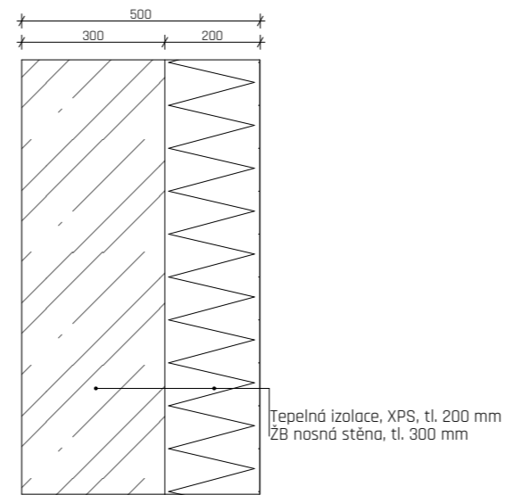
S2 OBVODOVÁ STĚNA POD TERÉNEM
