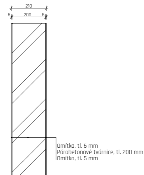
S6 PŘÍČKA
