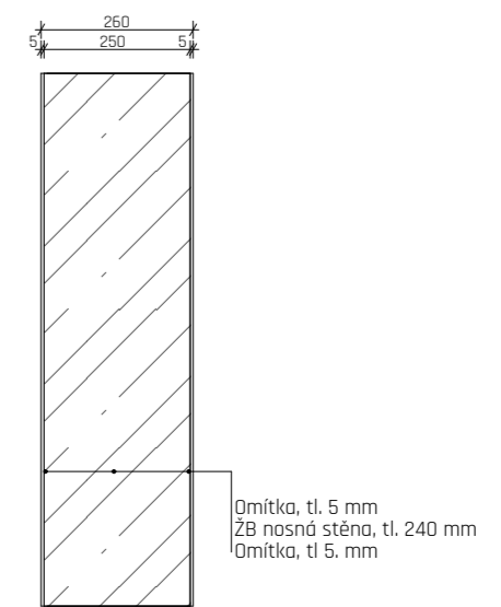
S4 VNITŘNÍ NOSNÁ STĚNA 250
