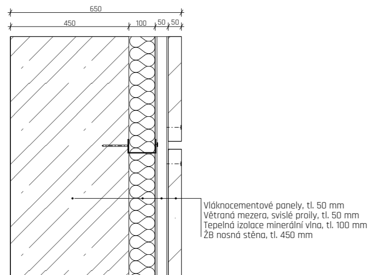
S7 OBVODOVÁ STĚNA K ULICI NAD TERÉNEM
