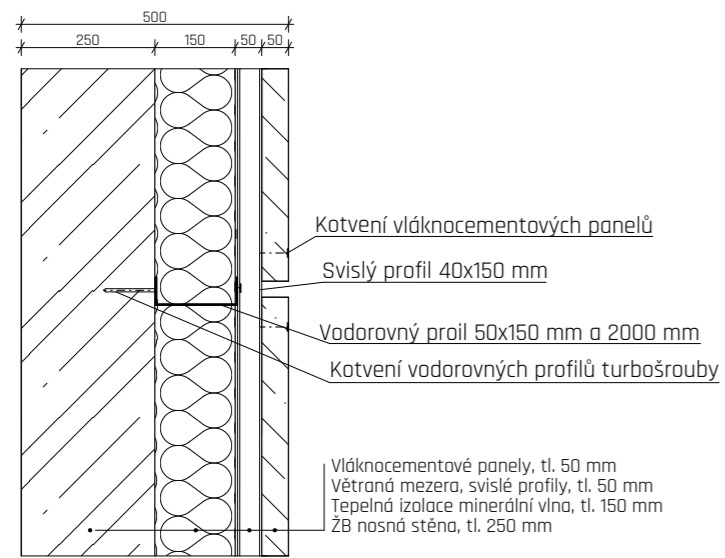
S1 OBVODOVÁ STĚNA NAD TERÉNEM
