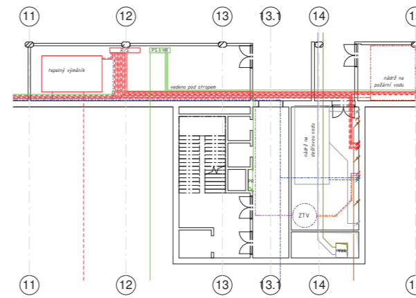
PŮDORYS IPP, CENTRÁLNÍ ČÁST S PŘÍPOJKAMI
