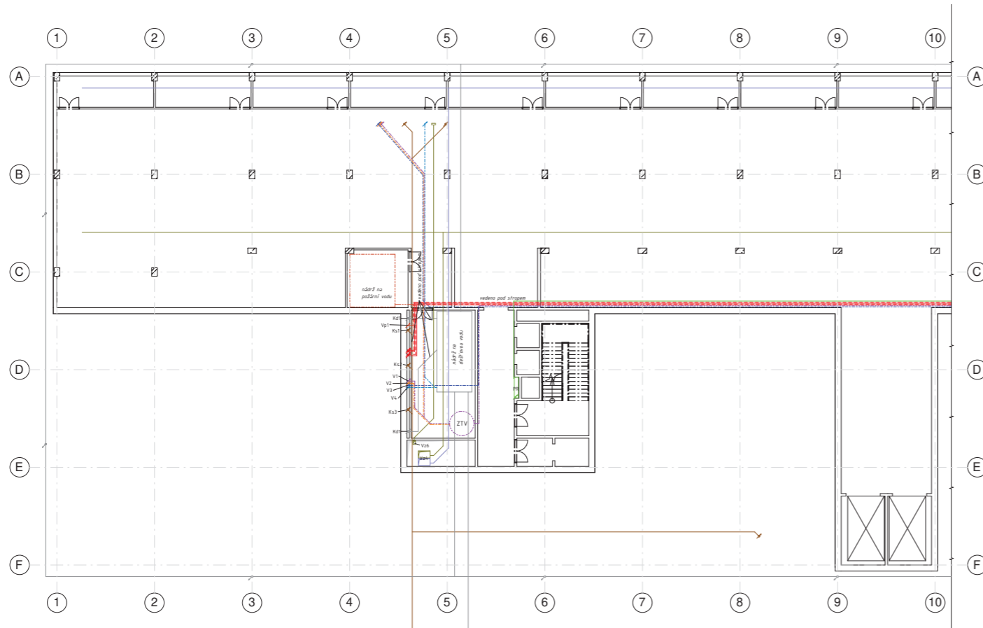
PŮDORYS IPP, ŘEŠENÁ ČÁST
