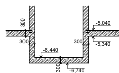
ŘEZ B-B
