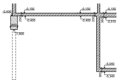
ŘEZ A-A
