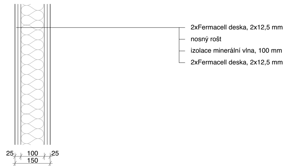
S05 SKLADBA VNITŘNÍ NENOSNÉ STĚNY, 150mm
