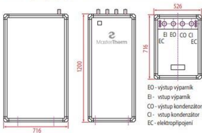
Rozměry a připojení modelů 22Z až 90Z:
