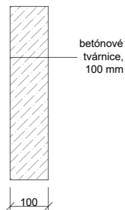
S9 Skladba vnútornej nenosnej priečky
