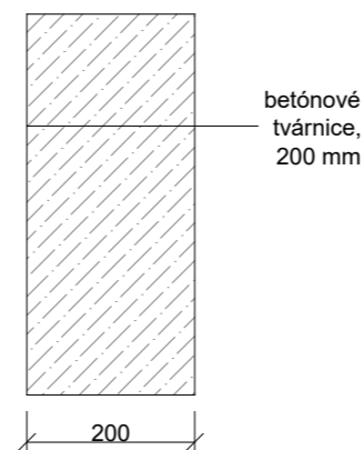
S10 Skladba medzibytovej nenosnej priečky
