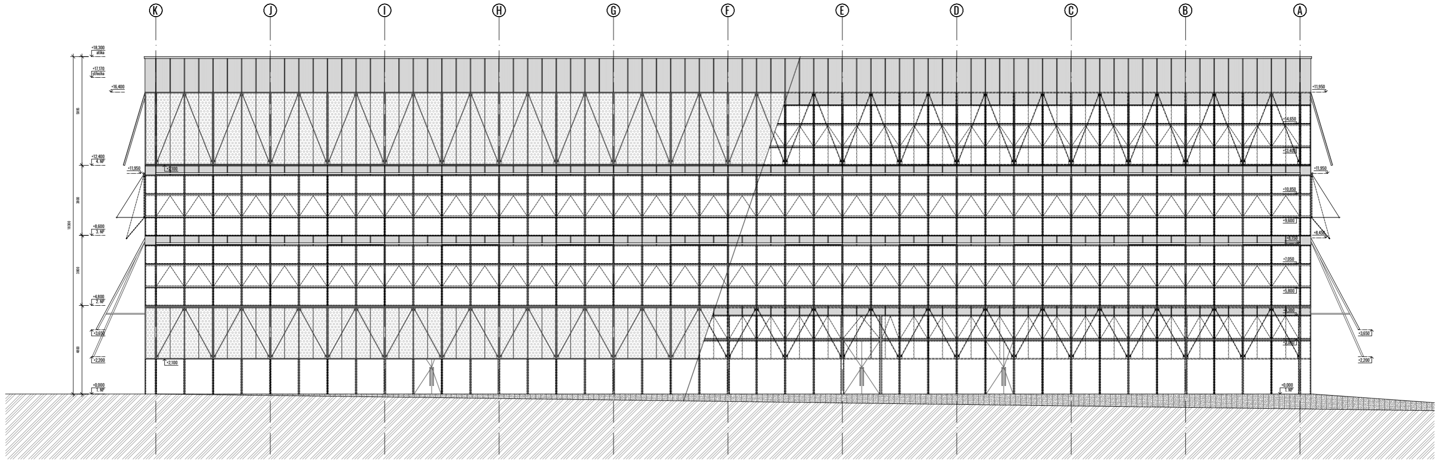
POHLED NA FASÁDNÍ PANELE
