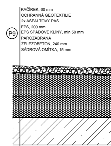
Střecha
