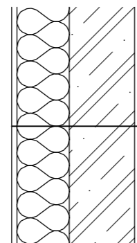
S1) Skladba - obvodová stěna
