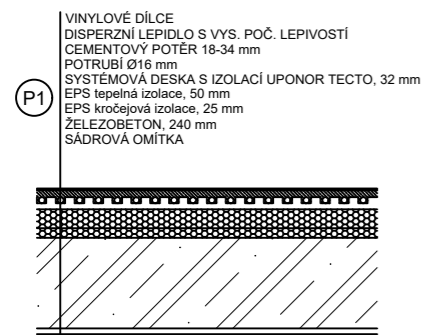
Podlaha - byt
