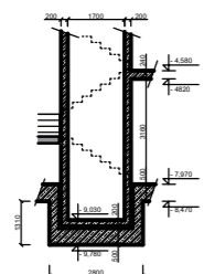
ŘEZ ZÁKLADEM VÝTAHOVÉ ŠACHTY B - B':
