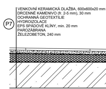
Podlaha nad stropní deskou garáže
