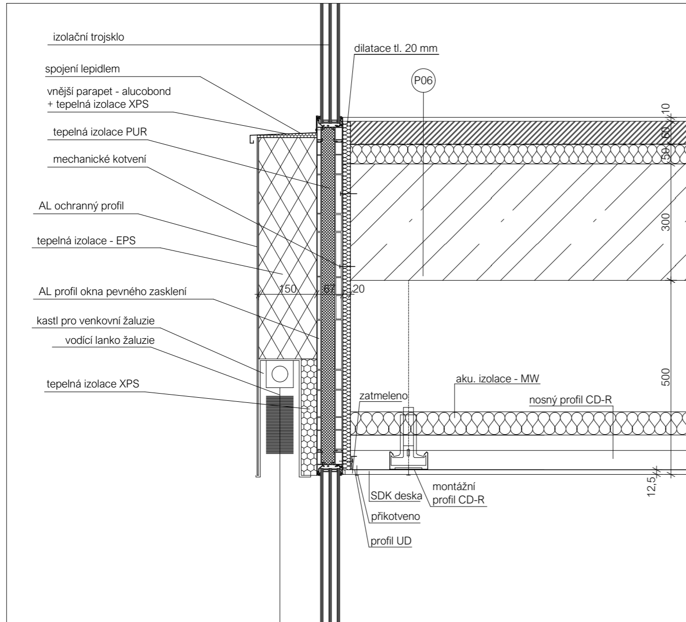
DETAIL Č. 5
