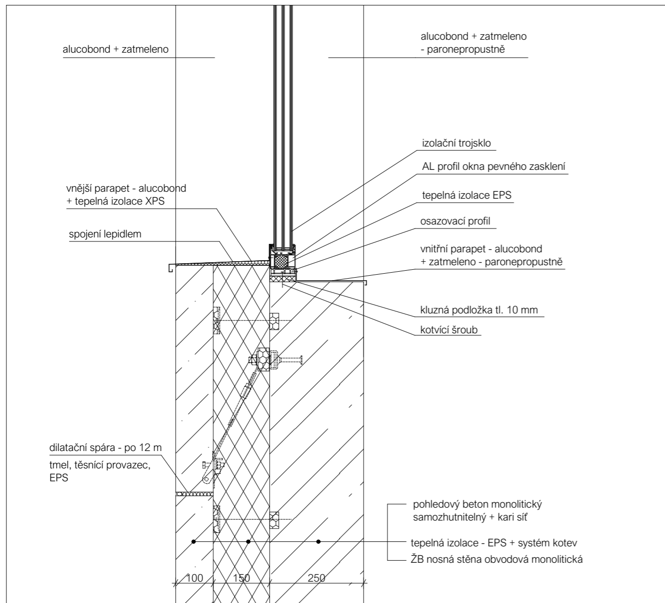
DETAIL Č. 7
