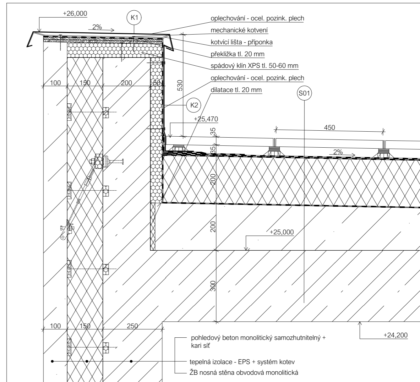
DETAIL Č. 4
