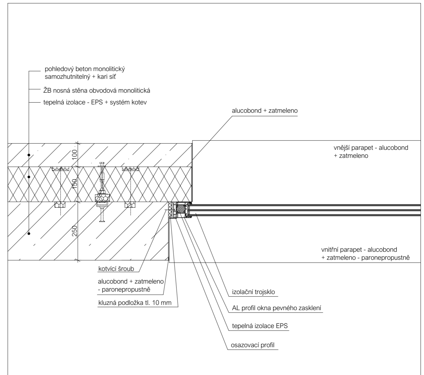
DETAIL Č. 8
