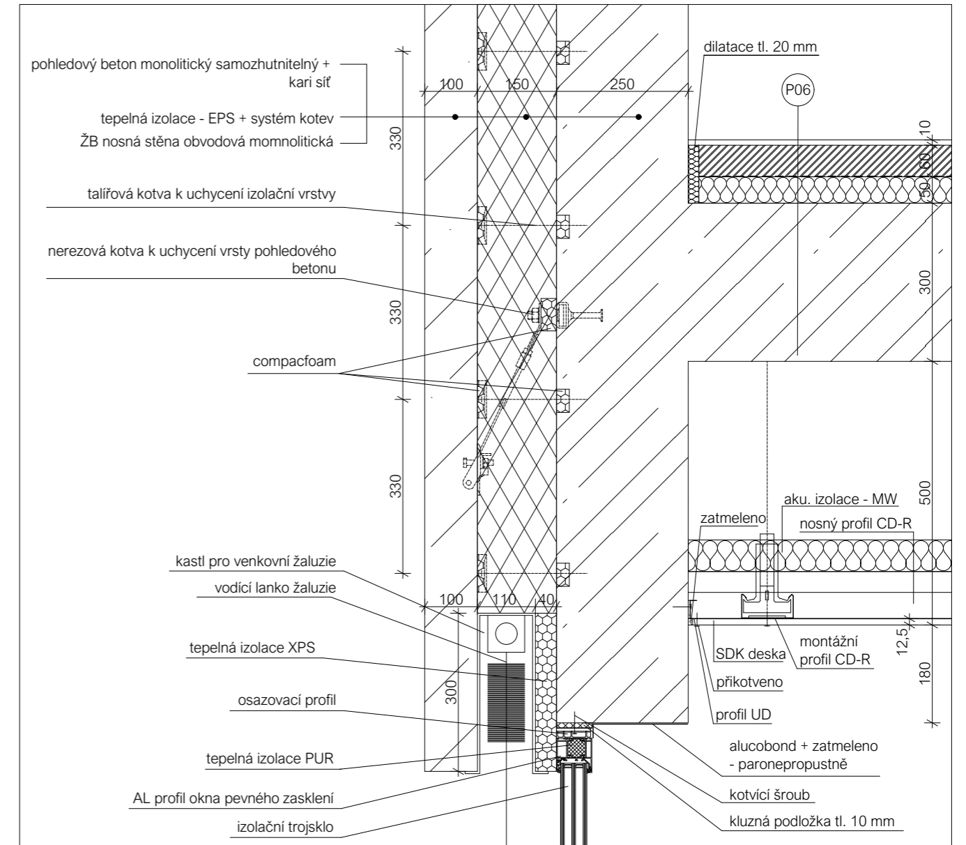
DETAIL Č. 6
