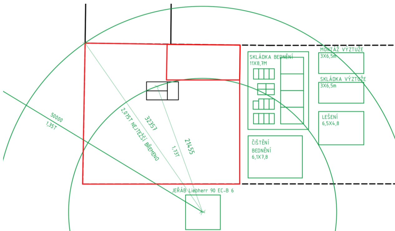
JEŘÁB Liebherr 90 EC-B 6
