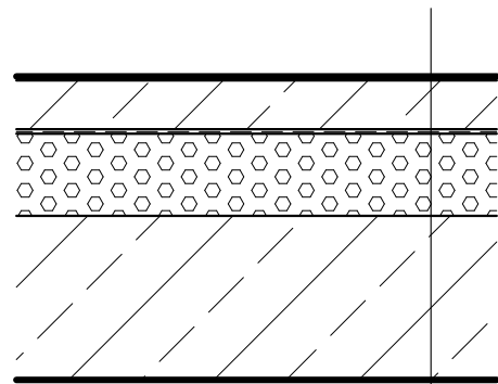
Podlaha společné prostory tl. 365mm
