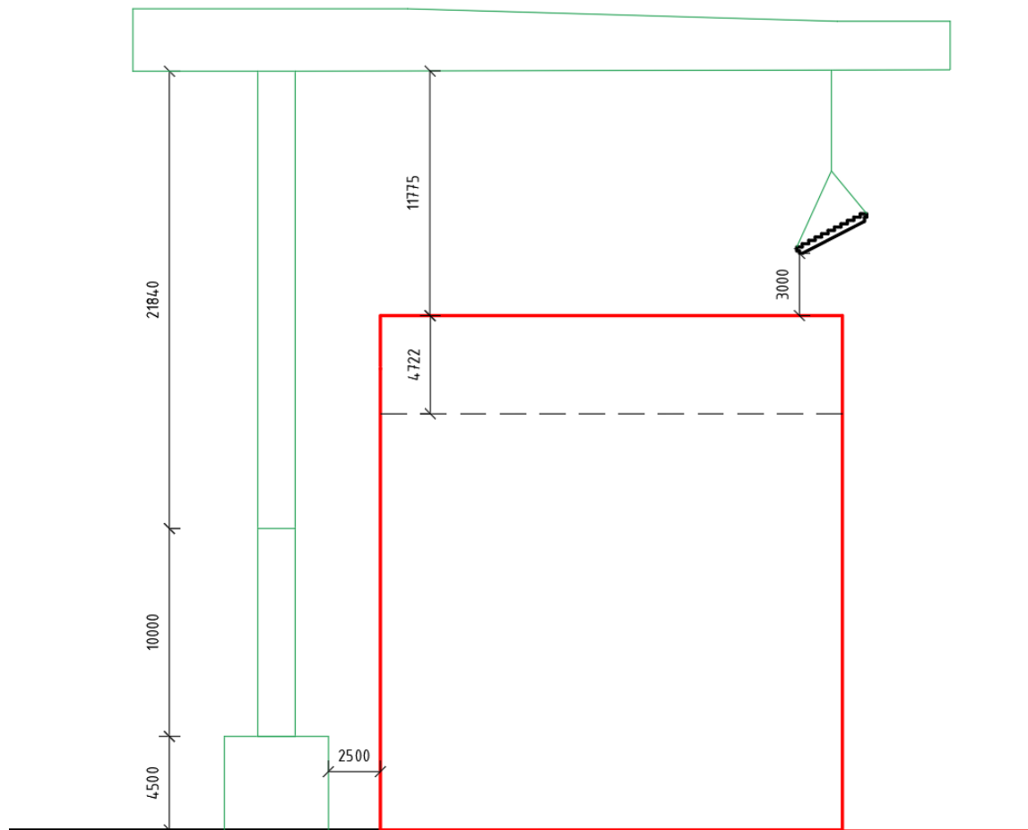
JEŘÁB Liebherr 90 EC-B 6
