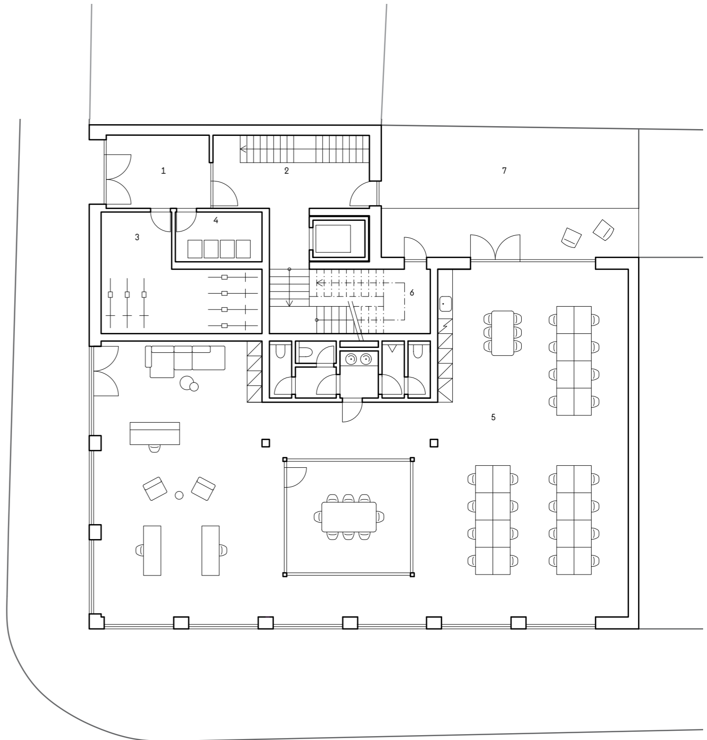
Půdorys 1.NP 1 zádveří 2 obslužné prostory 3 kolárně 4 odpad 5 prostor parteru 6 skladovací prostor 7 dvůr
