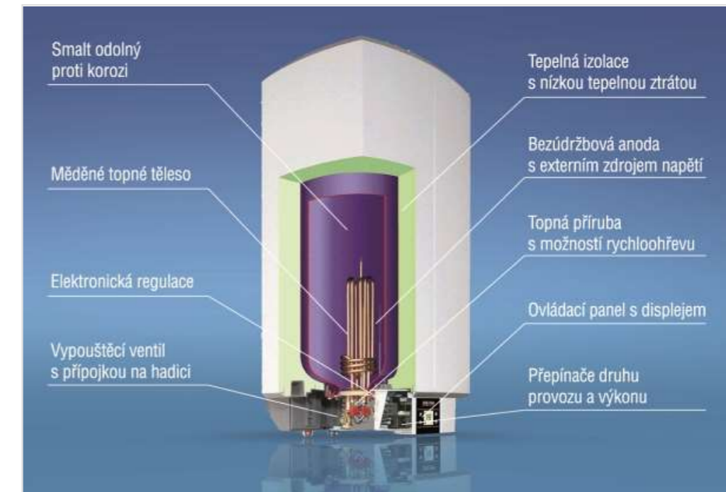
Popis bojleru v řezu
