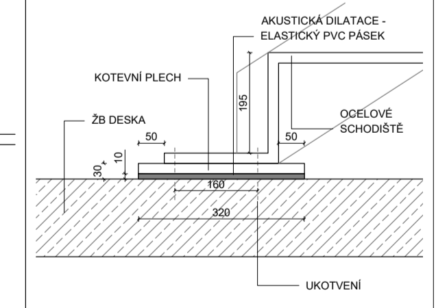
DETAIL ÚLOŽENÍ OC. SCHOD. NA DESKU V2
