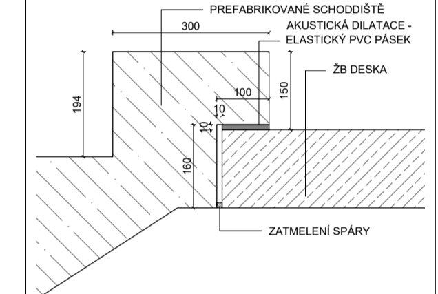
DETAIL ÚLOŽENÍ ŽB SCHOD. NA DESKU V3
