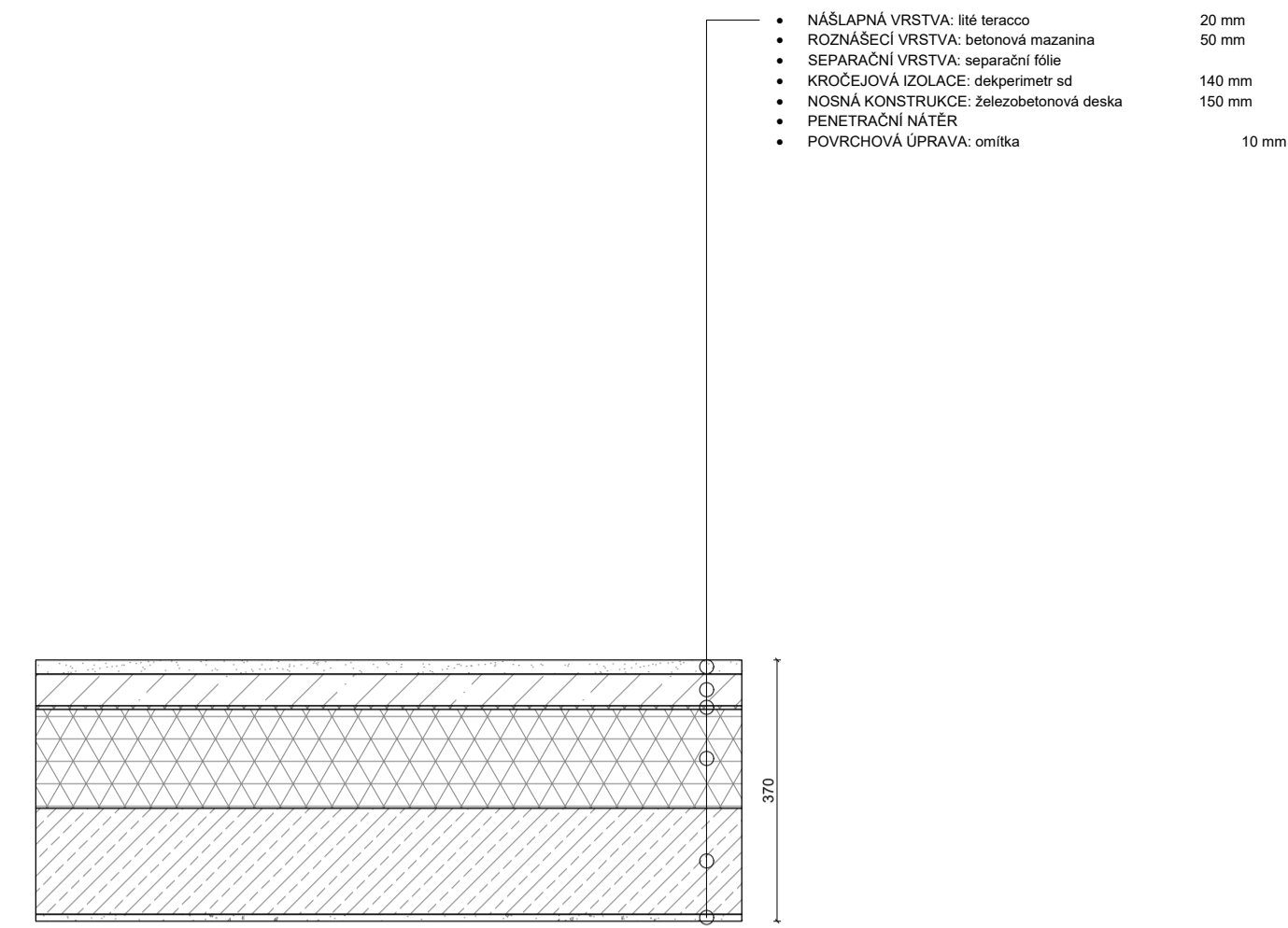
P7. SKLADBA PODLAHY NAD EXTERIÉREM
