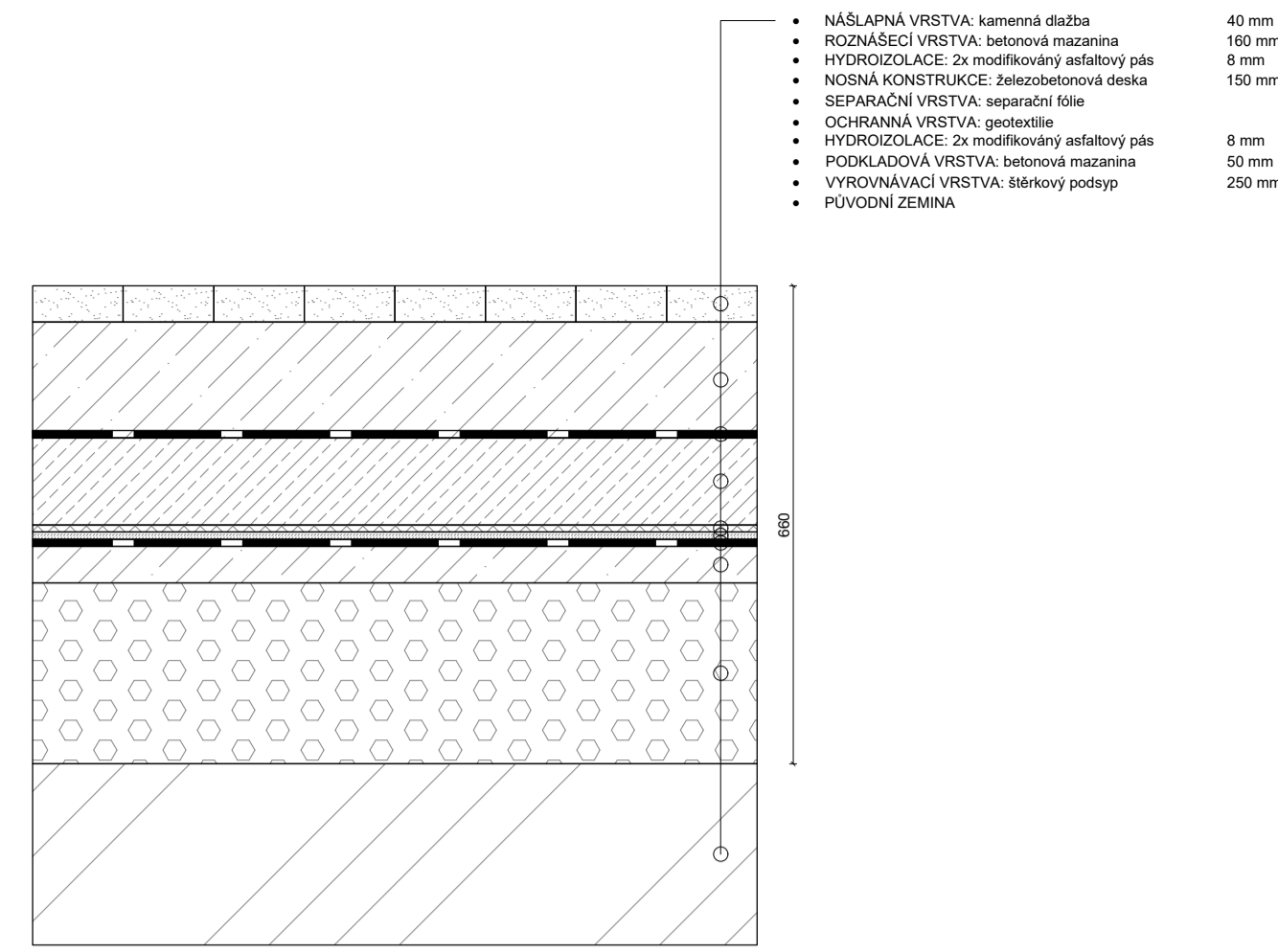
P6. SKLADBA PODLAHY WC NA TERÉNU
