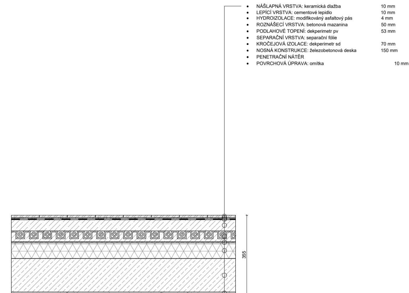
P11. SKLADBA PODLAHY WC S PODLAHOVÝM TOPENÍM
