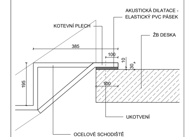
DETAIL ÚLOŽENÍ OC. SCHOD. NA DESKU V2
