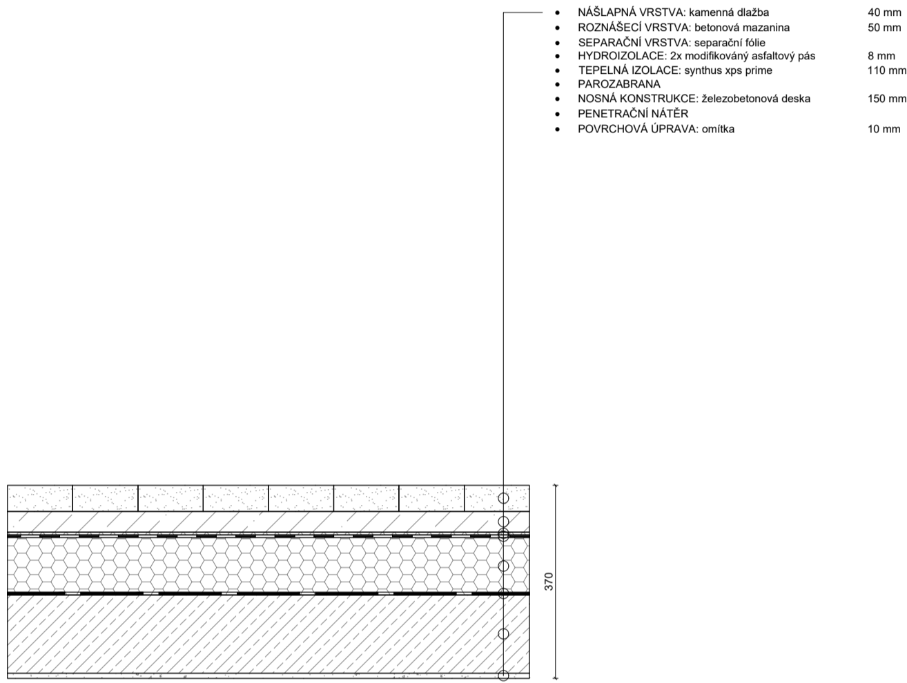
P9. SKLADBA PODLAHY WC NAD VÝTAPĚNÝM PROSTOREM
