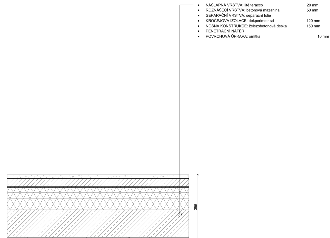
P13. SKLADBA PODLAHY PODESTY V2
