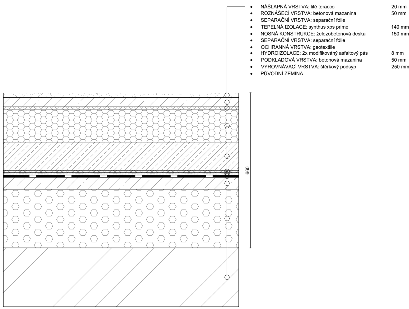
P5. SKLADBA CHODNÍKU NAD SUTERÉNEM
