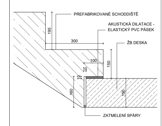
DETAIL ÚLOŽENÍ ŽB SCHOD. NA DESKU V2
