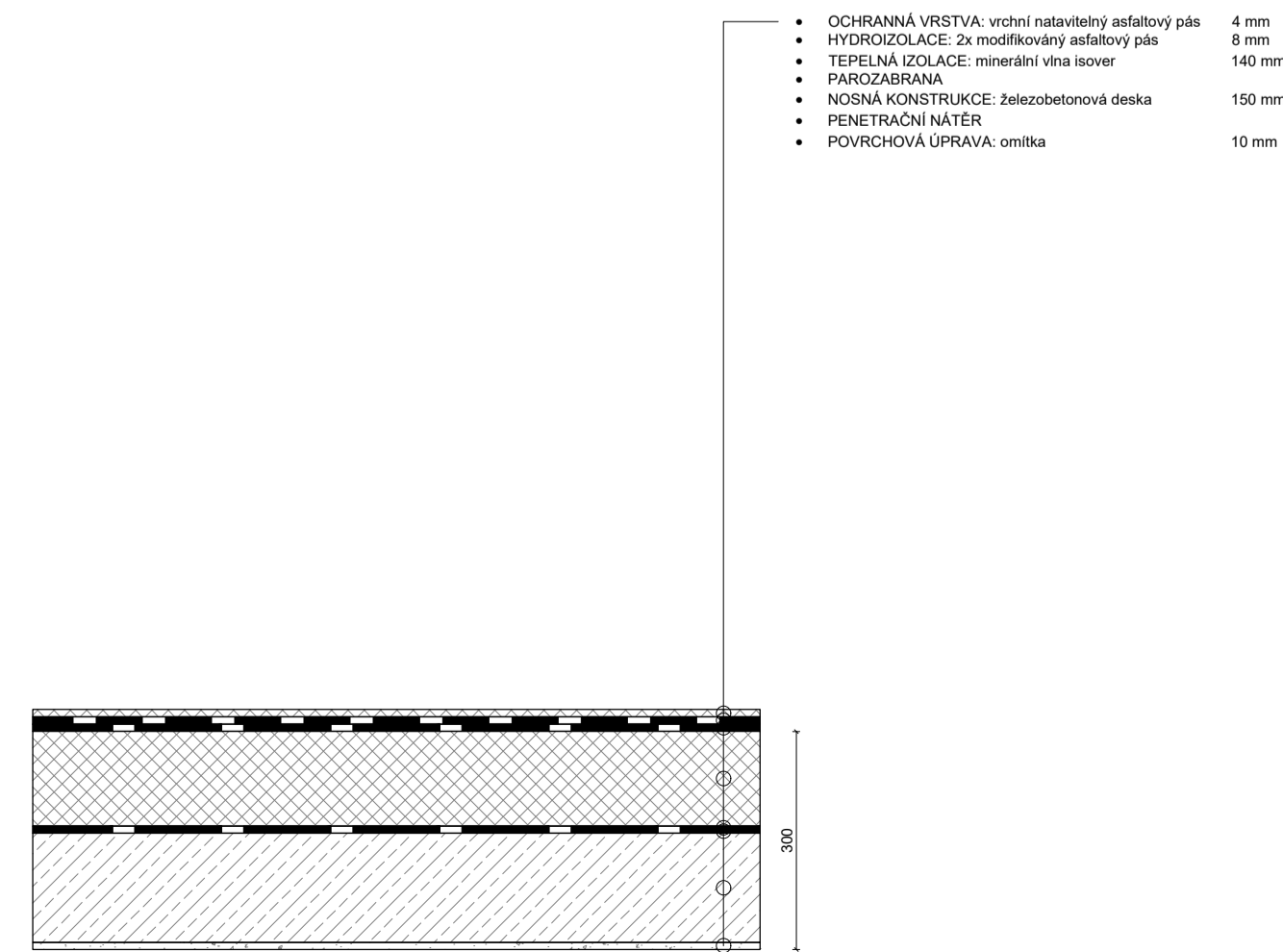
S2. SKLADBA STŘECHY V2
