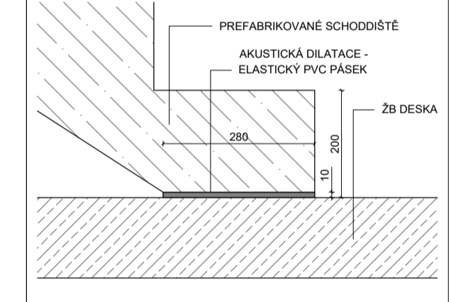
DETAIL ÚLOŽENÍ OC. SCHOD. NA DESKU V1
