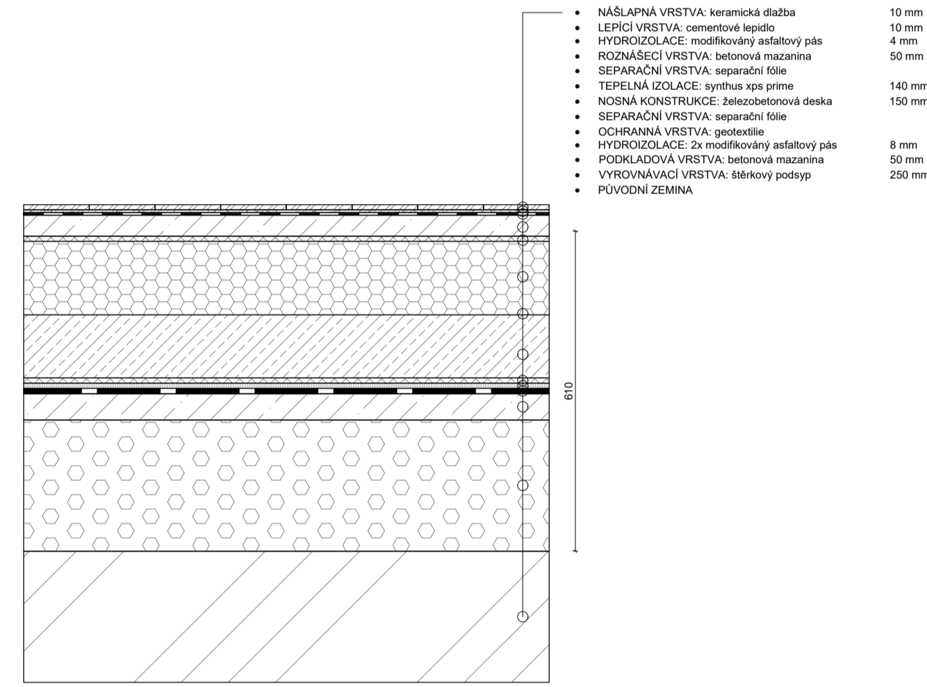
P10. SKLADBA PODLAHY S PODLAHOVÝM TOPENÍM
