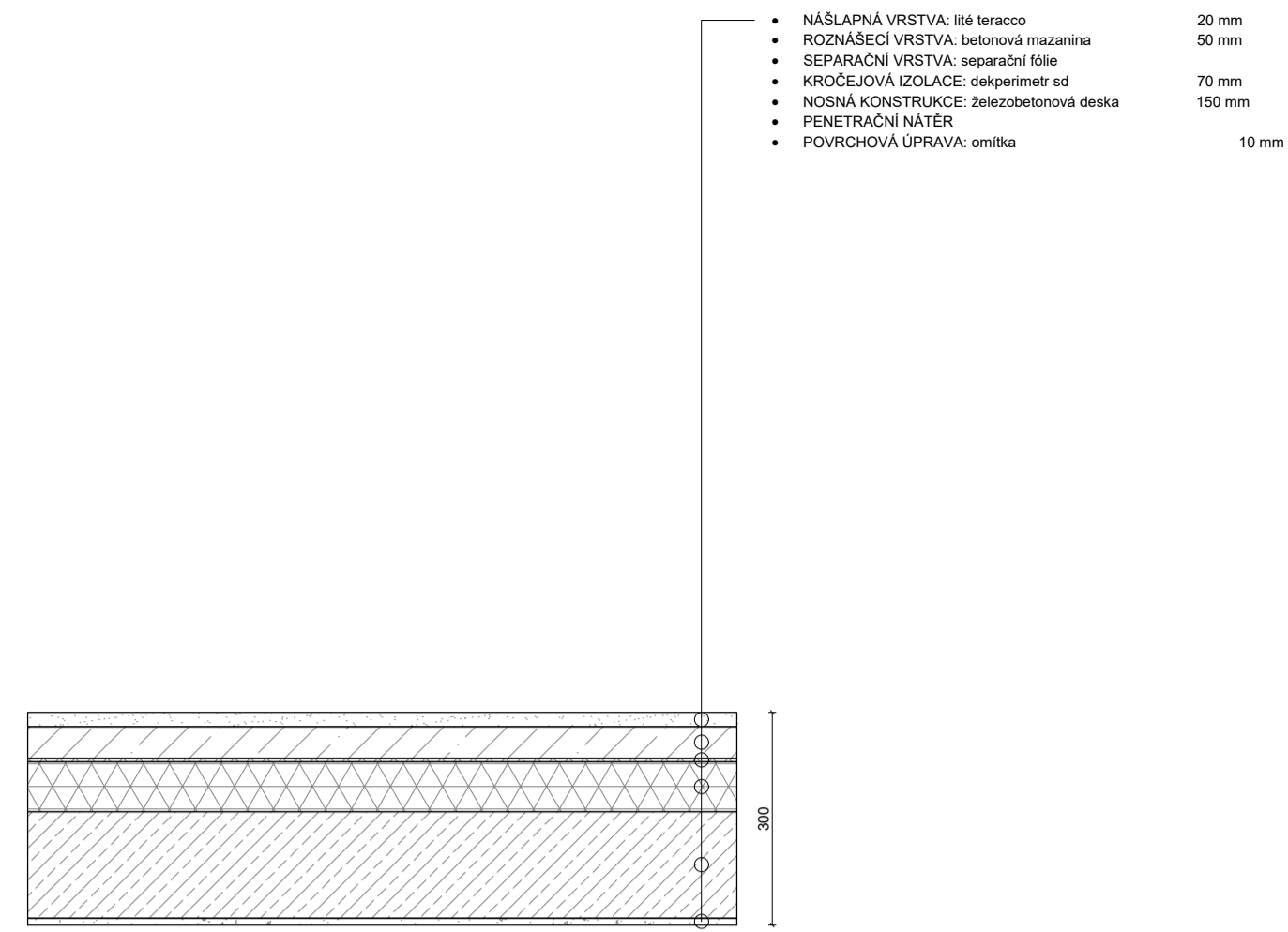
P12. SKLADBA PODLAHY LODŽIE
