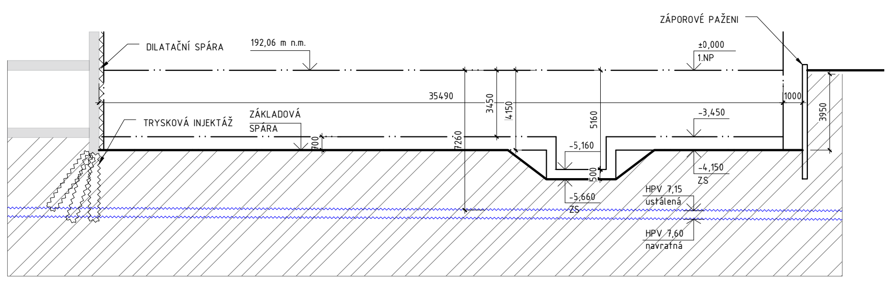
ŘEZ A-A
