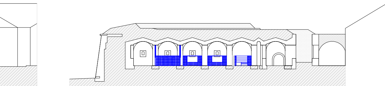
pozdĺžny rez kasematami
