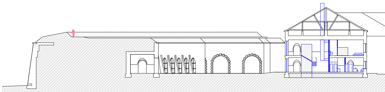
priečny rez
