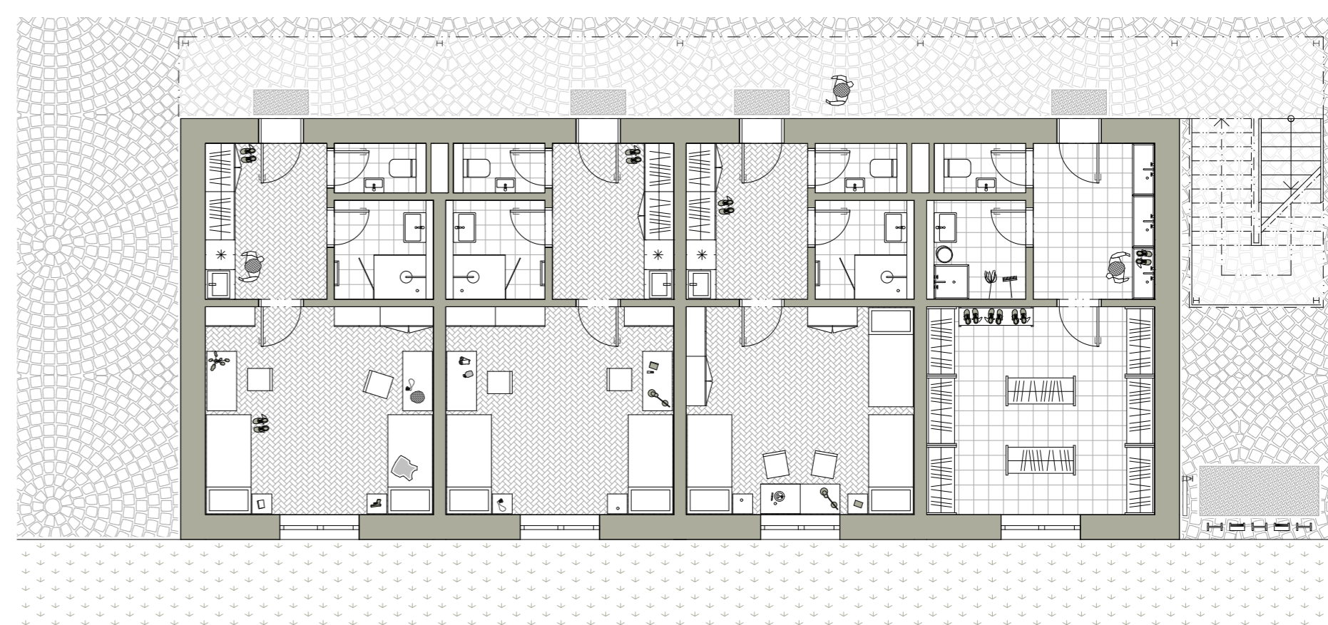
půdorys 1 np, m 1:75
