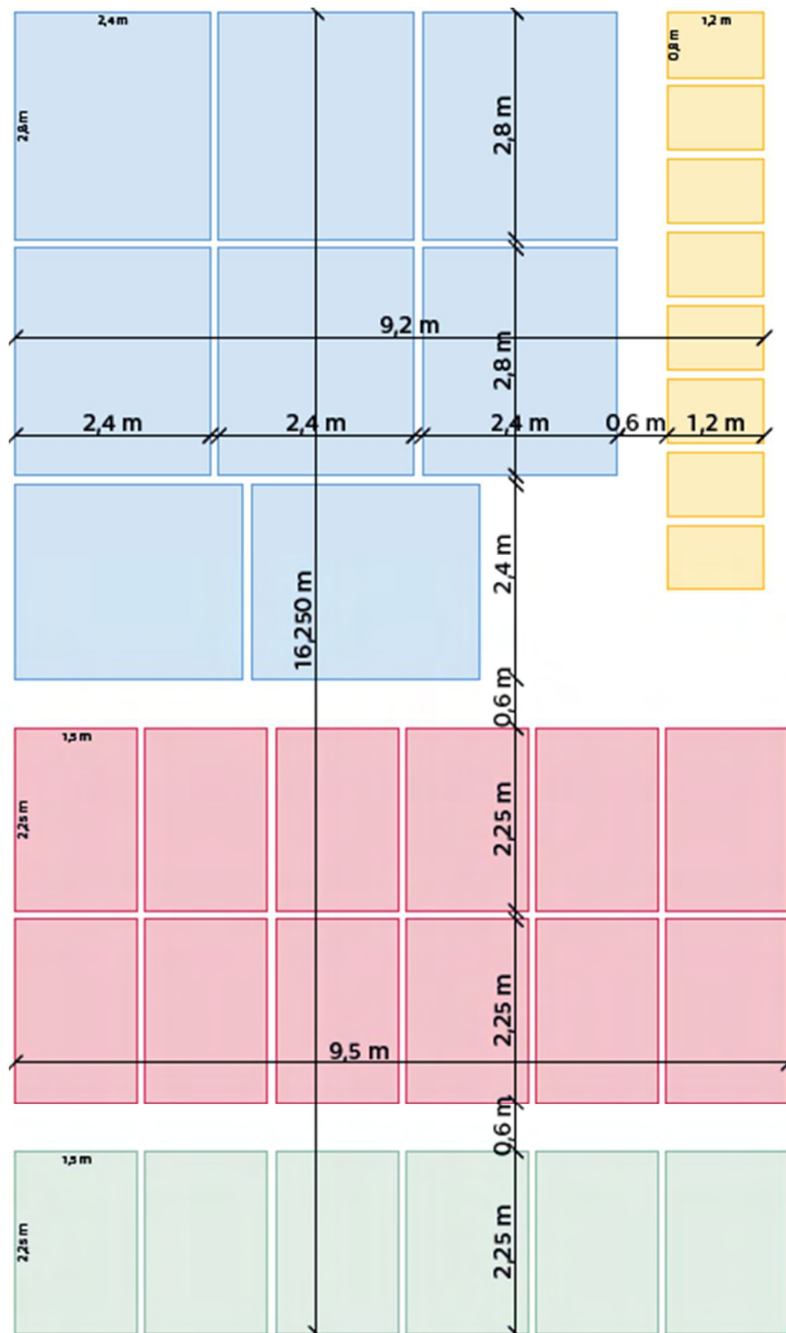
Obrázek 4: schéma pomocných konstrukcí
