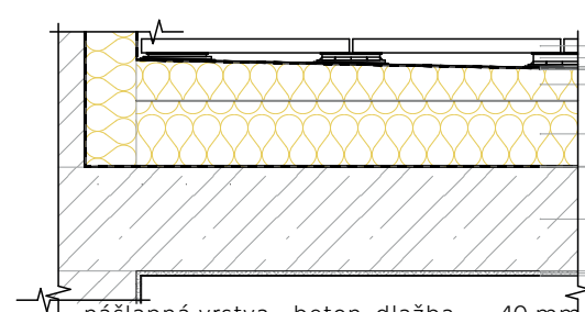
ST03 - pochozí střecha - terasa v 7. NP
