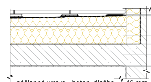
ST04 - "předzahrádky" nad garážemi
