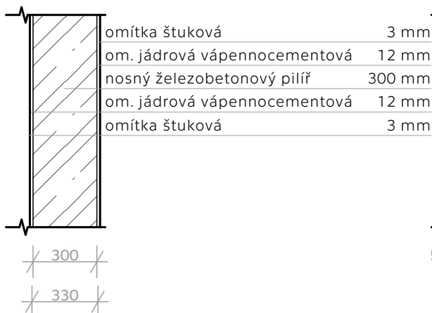
S06 - ŽB nosné sloupky v 5. NP - 10. NP
