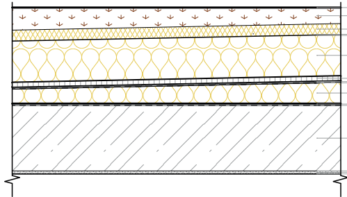
ST01 - vegetační střecha
