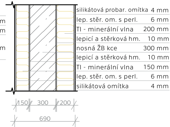
S05 - zateplená stěna ve skladu odpadu
