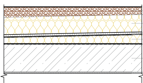
ST02 - střecha s kačírkem
