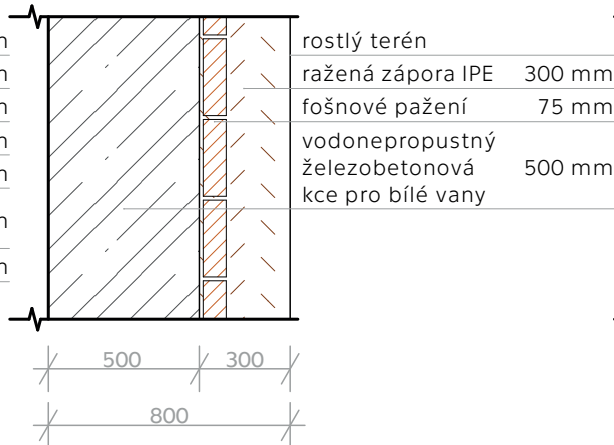
S04 - obvodová stěna v kontaktu s terénem
