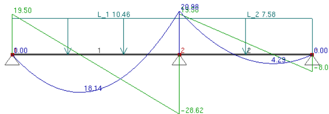
Obr. 5 – Návrh stropní desky, varianta B
