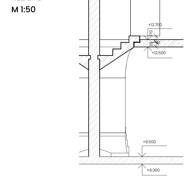
SCHODIŠTĚ_C: ŘEZ B-B' M 1:50
