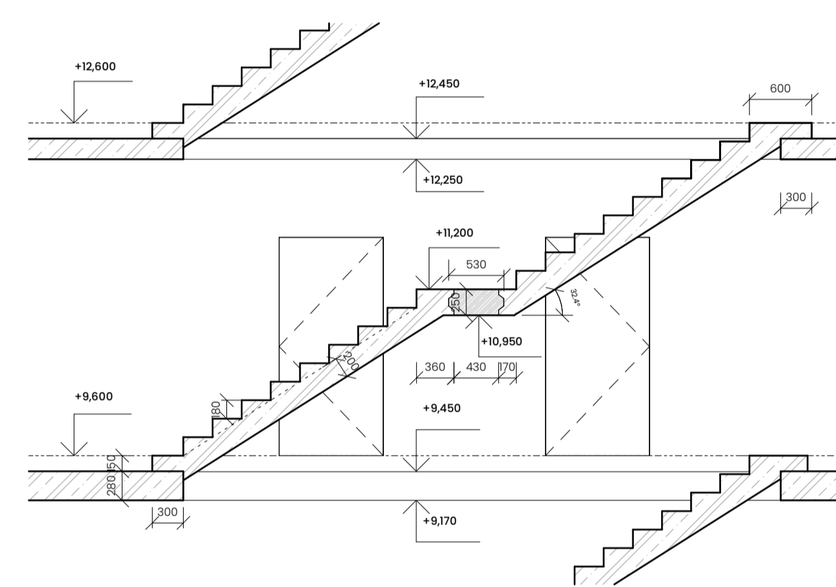
ŘEZ A-A' M 1:50
