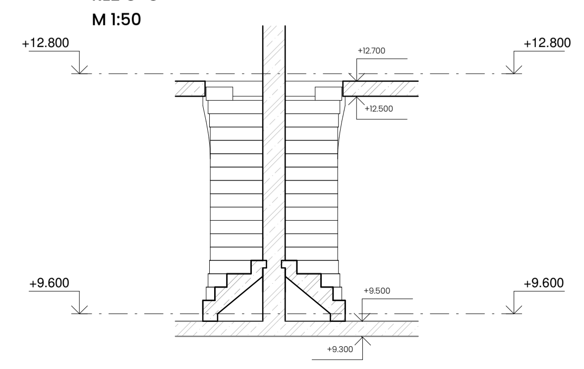
SCHODIŠTĚ_C: ŘEZ C-C' M 1:50
