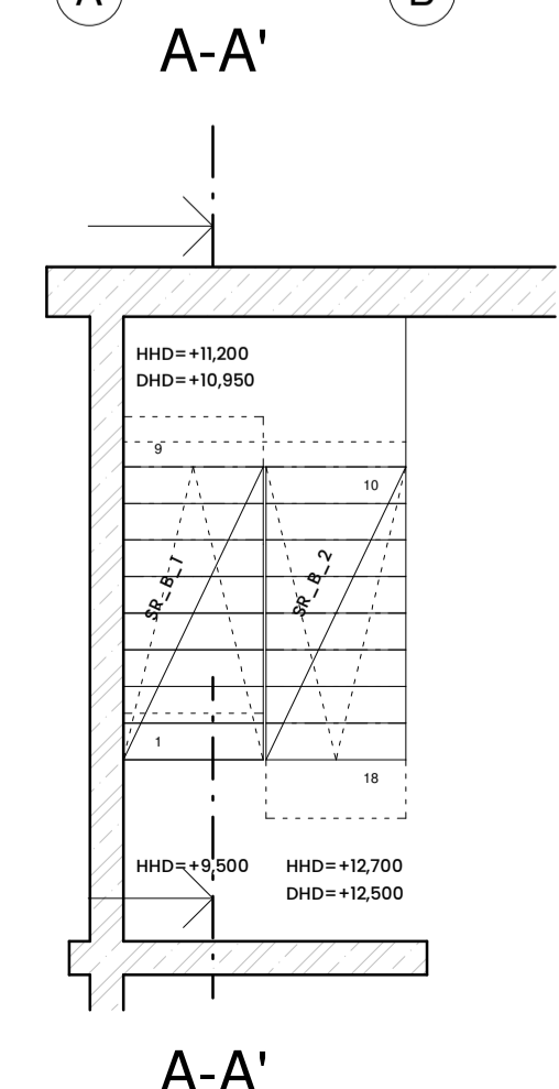
SCHODIŠTĚ_B M 1:50
