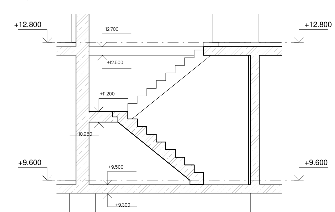
SCHODIŠTĚ_B: ŘEZ A-A' M 1:50
