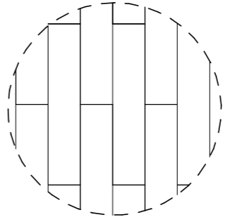
Schéma kladenia vinylovej podlahy
