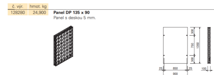
Obr. 5 – Panel debnenia 135x90mm
