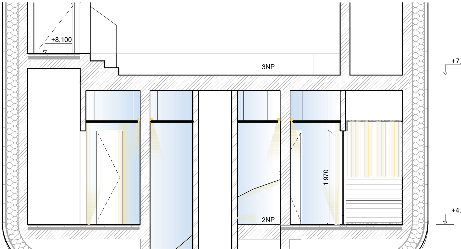
ŘEZ
