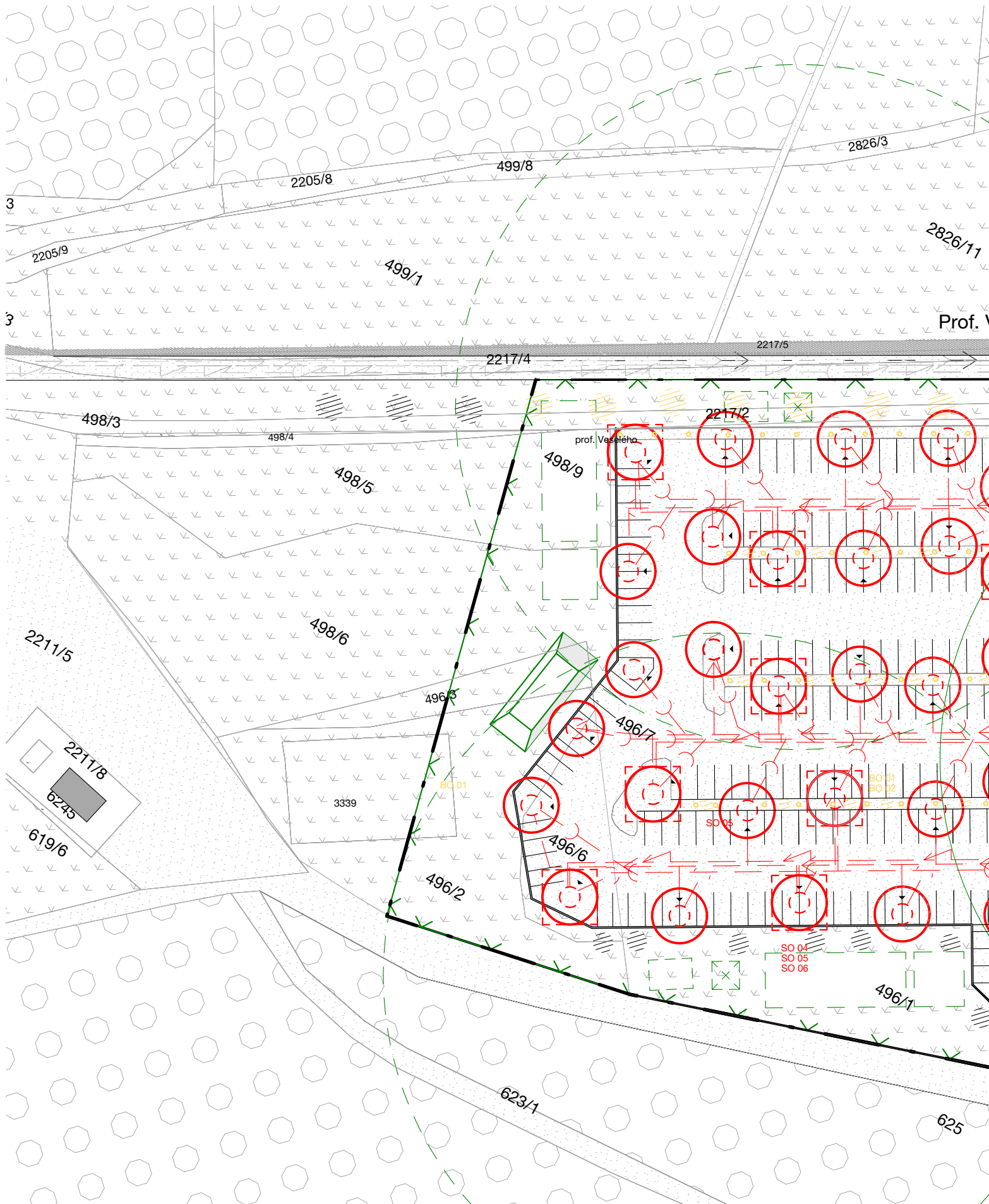
WELLNESS A HOTEL - GLASSFUL-L KOORDINAČNÍ SITUAČNÍ VÝKRES
