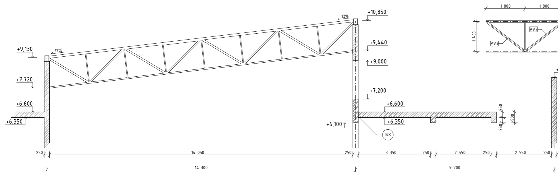
ŘEZ B-B'
