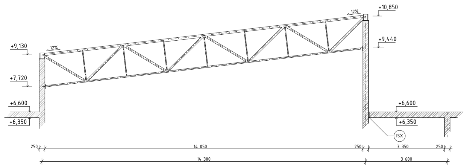
ŘEZ A-A'
