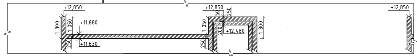
ŘEZ A-A'
