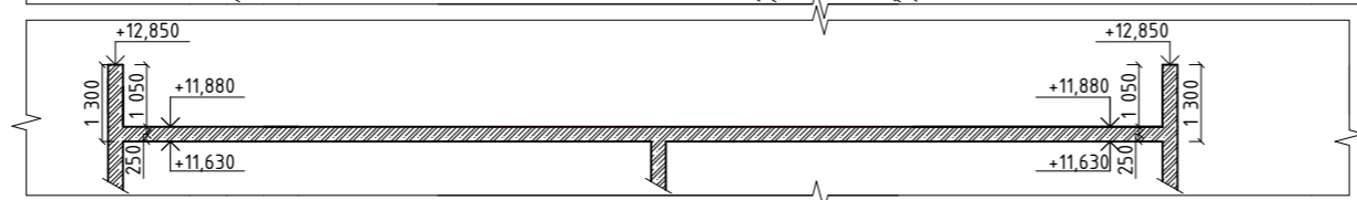
ŘEZ D-D'
