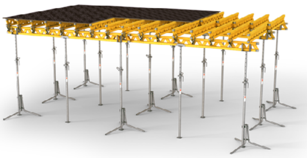
Peri MULTIFLEX
