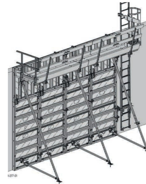
Obrázek 3: Bednění stěn Framax Xlife, zdroj: www.doka.com
