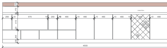
POHLED C-C'
