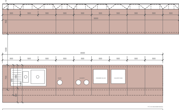
PŮDORYS
