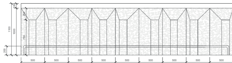
POHLED C-C'
