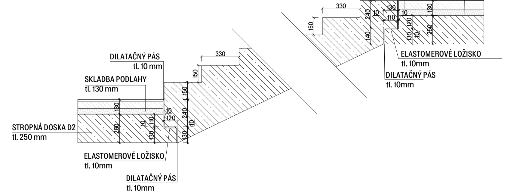
DETAIL ULOŽENIA SCHODISKOVÉHO RAMENA SR1 M 1:20
