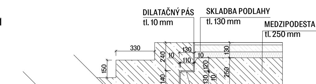
DETAIL ULOŽENIA SCHODISKOVÉHO RAMENA SR1 M 1:20
