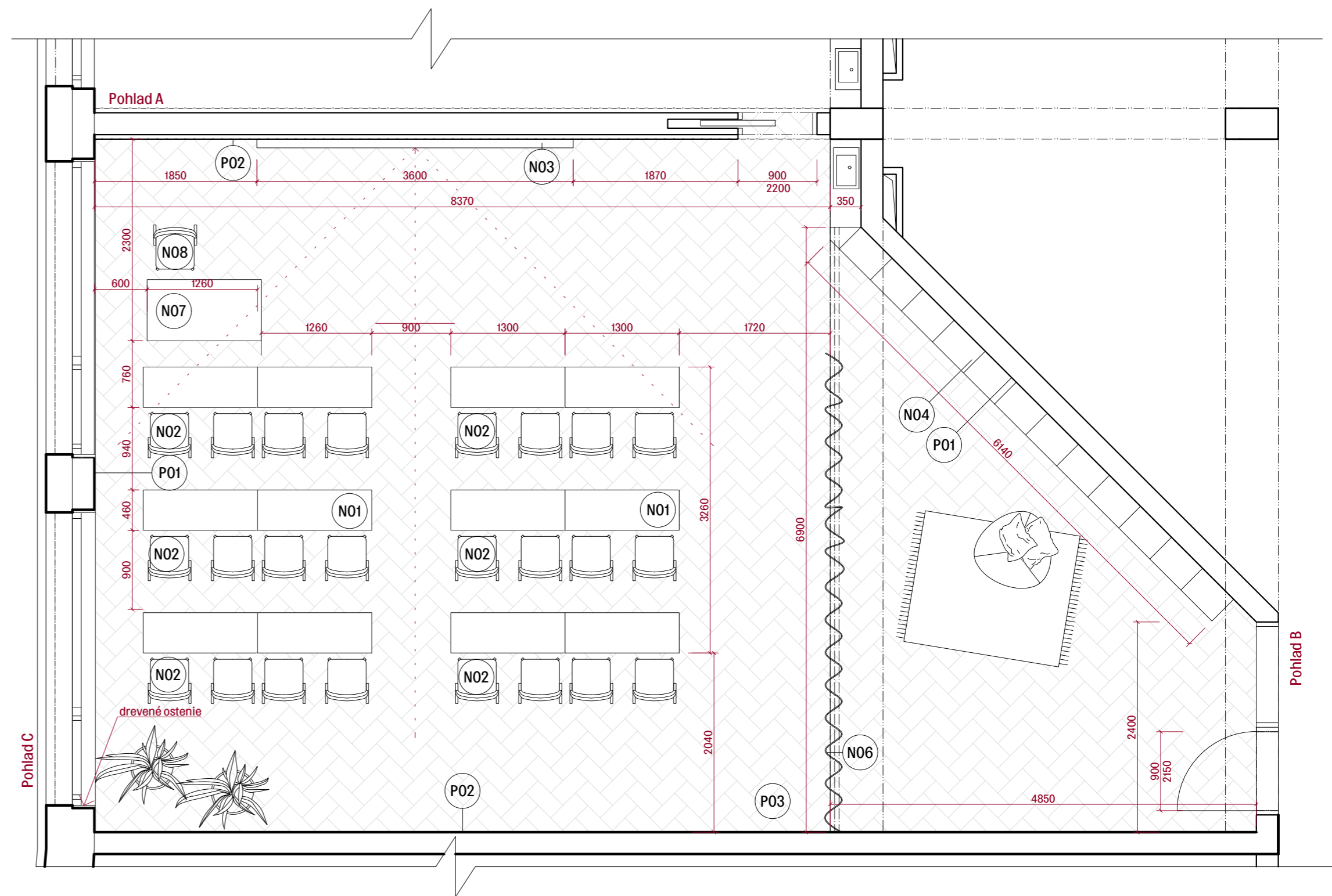
PÔDORYS TRIEDY 2.12
