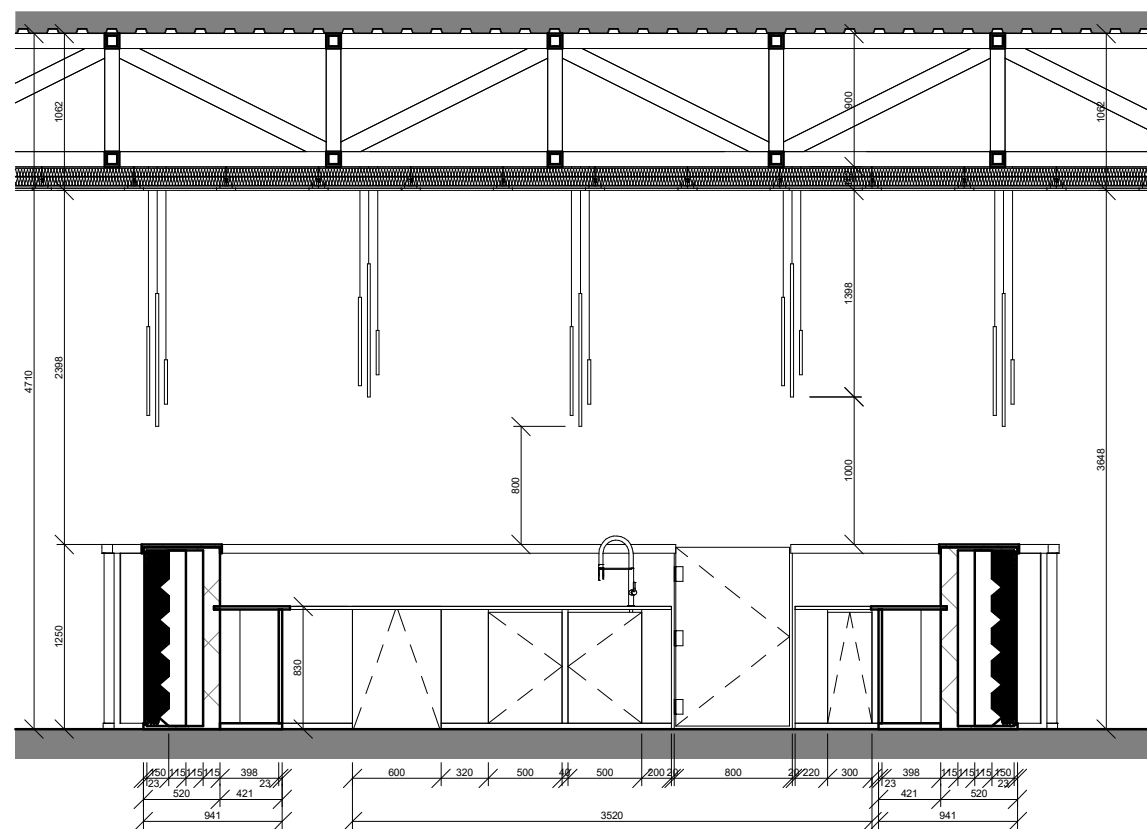
POHLED B 1:50
