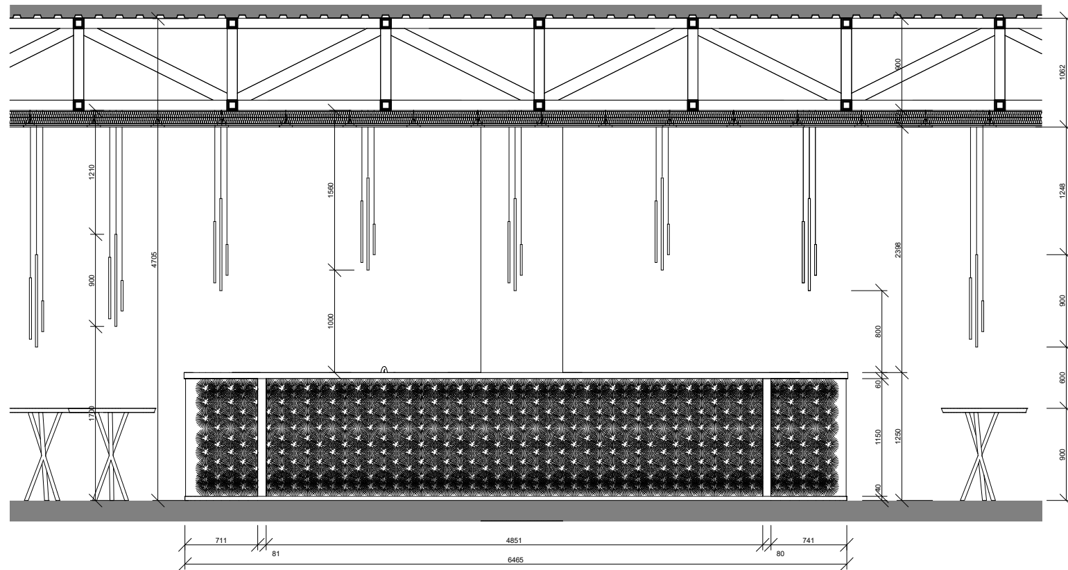
POHLED A 1:50
