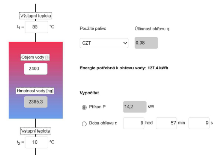
Bilance zdroje tepla
