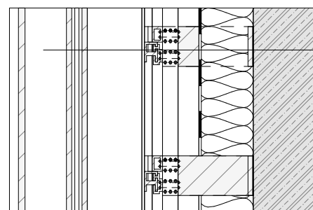
S02 OBVODOVÁ NOSNÁ STĚNA
