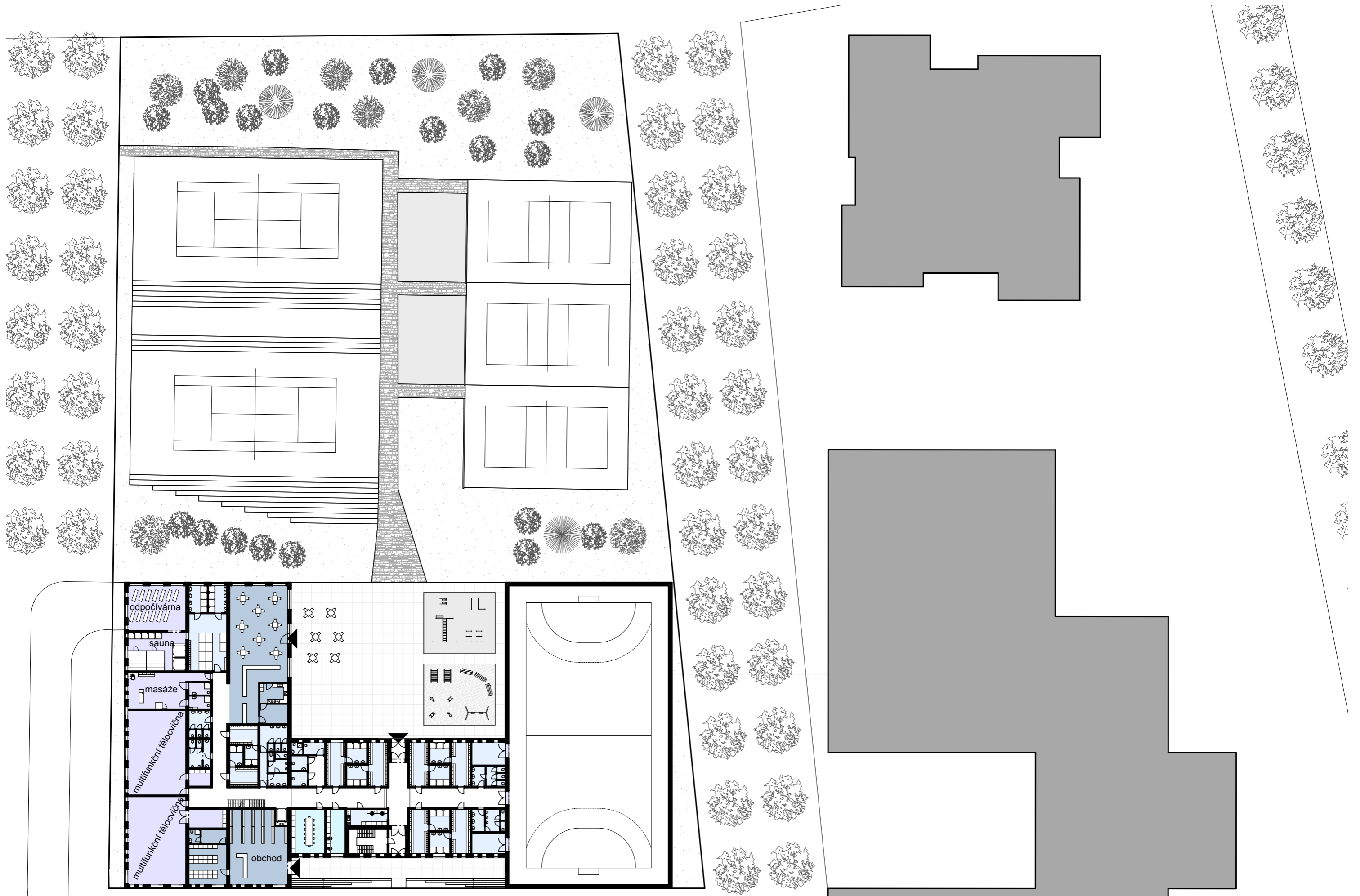
SITUACE POZEMKU, 1:500
