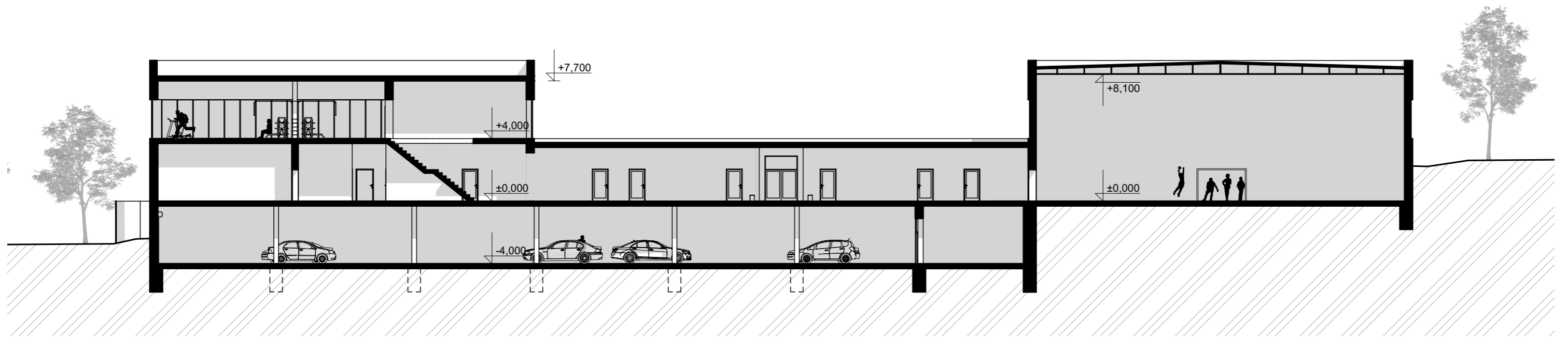
PODÉLNÝ ŘEZ, 1:250
