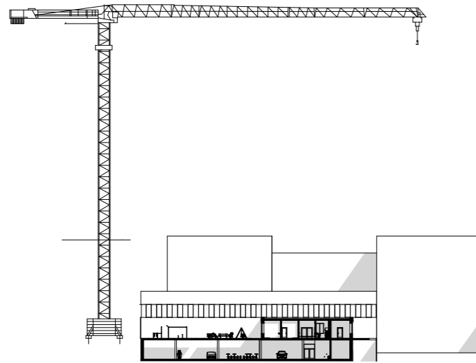
Schéma výšky jeřábu
