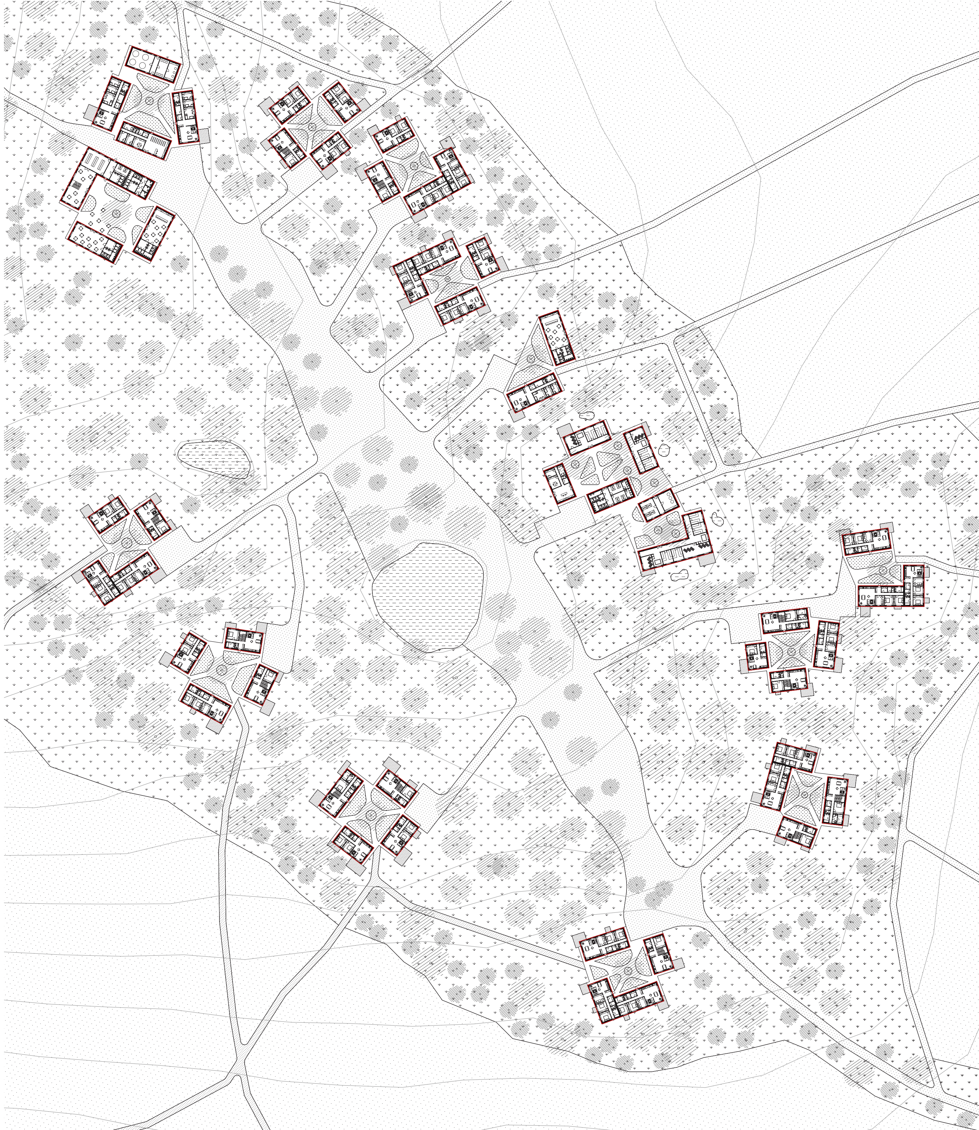
„Situace parteru“ Oldřichov návrh, M 1:800
