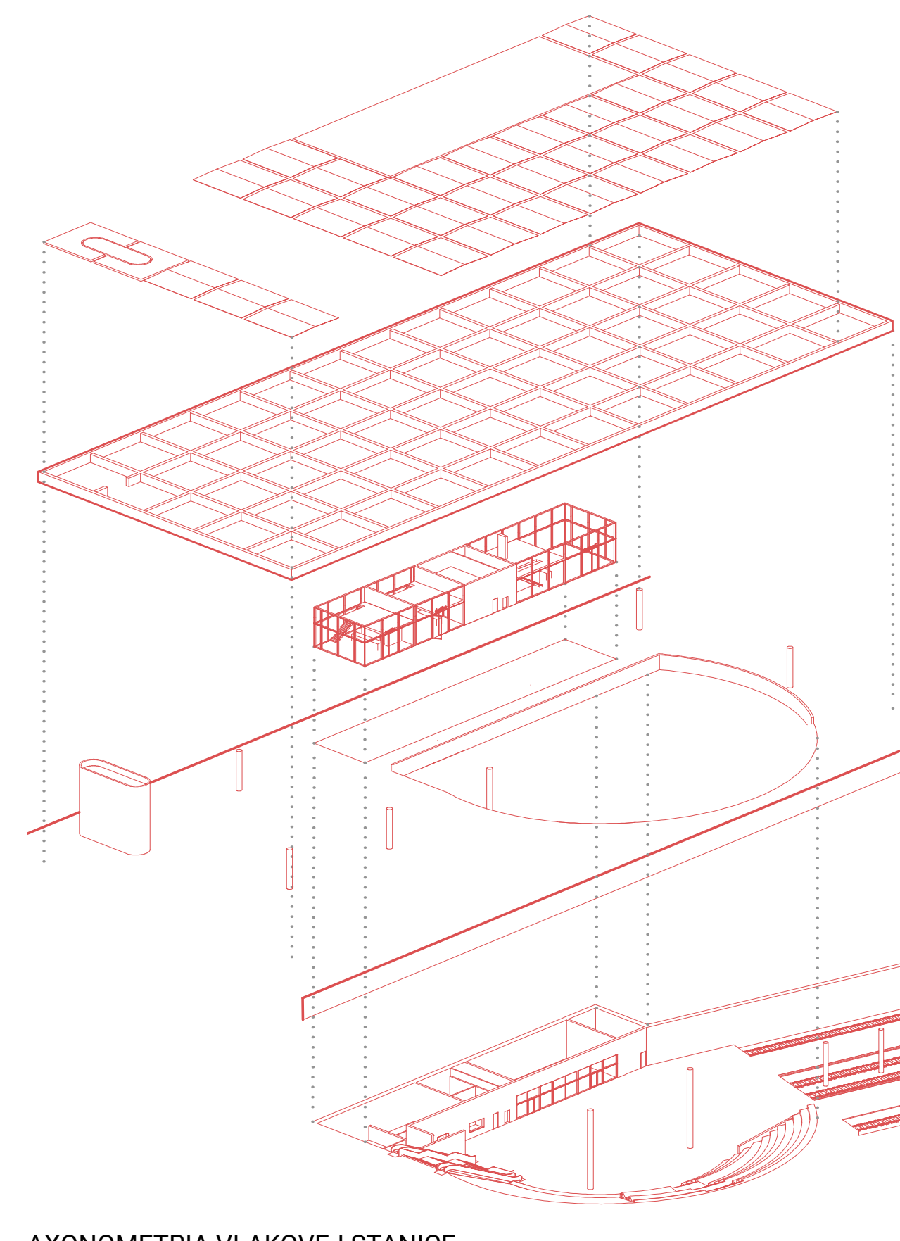
AXONOMETRIA VLAKOVEJ STANICE
