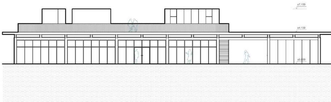
Pohľad severozápadný M 1:250
