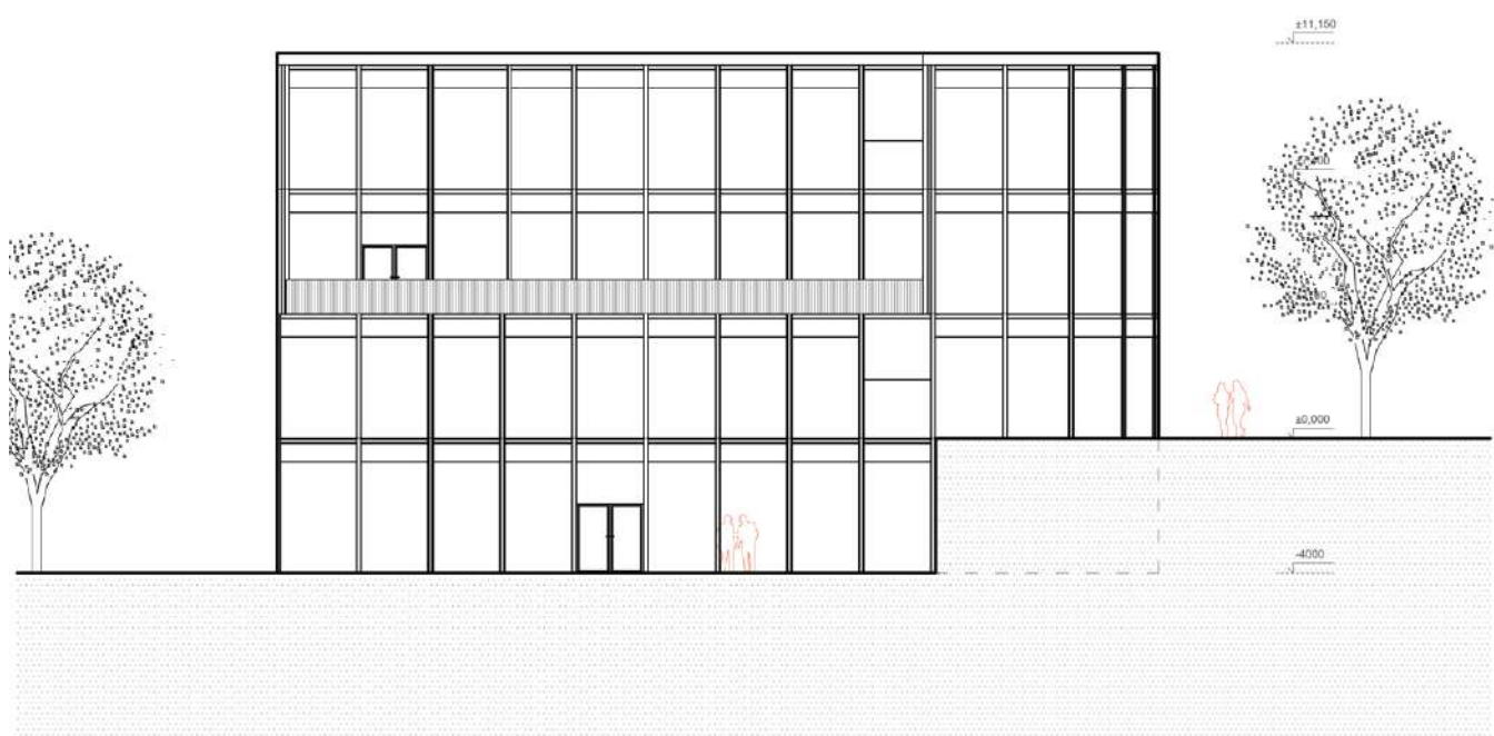
Pohľad juhozápadný M 1:250
