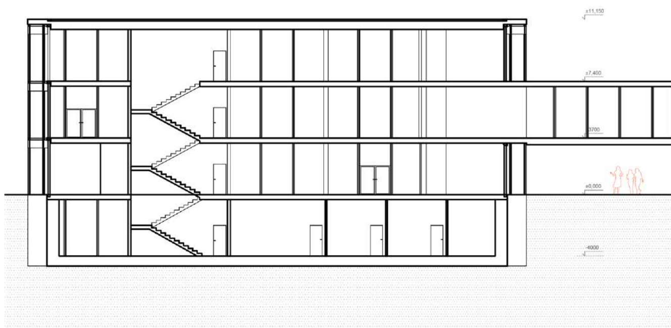
Rez pozdĺžný M 1:250
