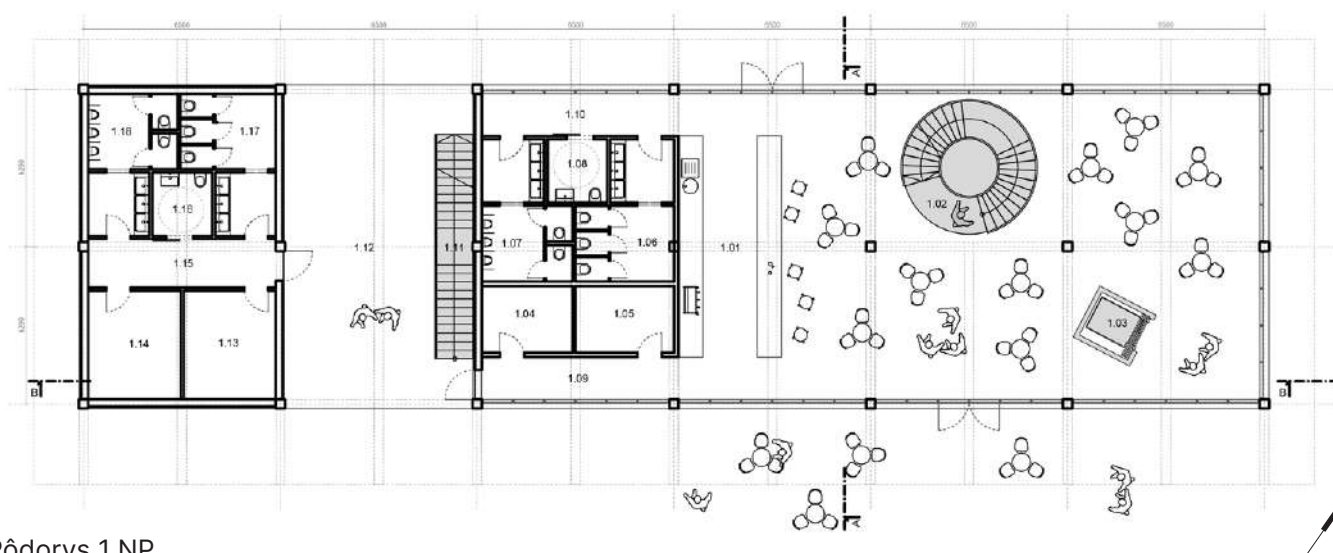
Pôdorys 1.NP M 1:250
