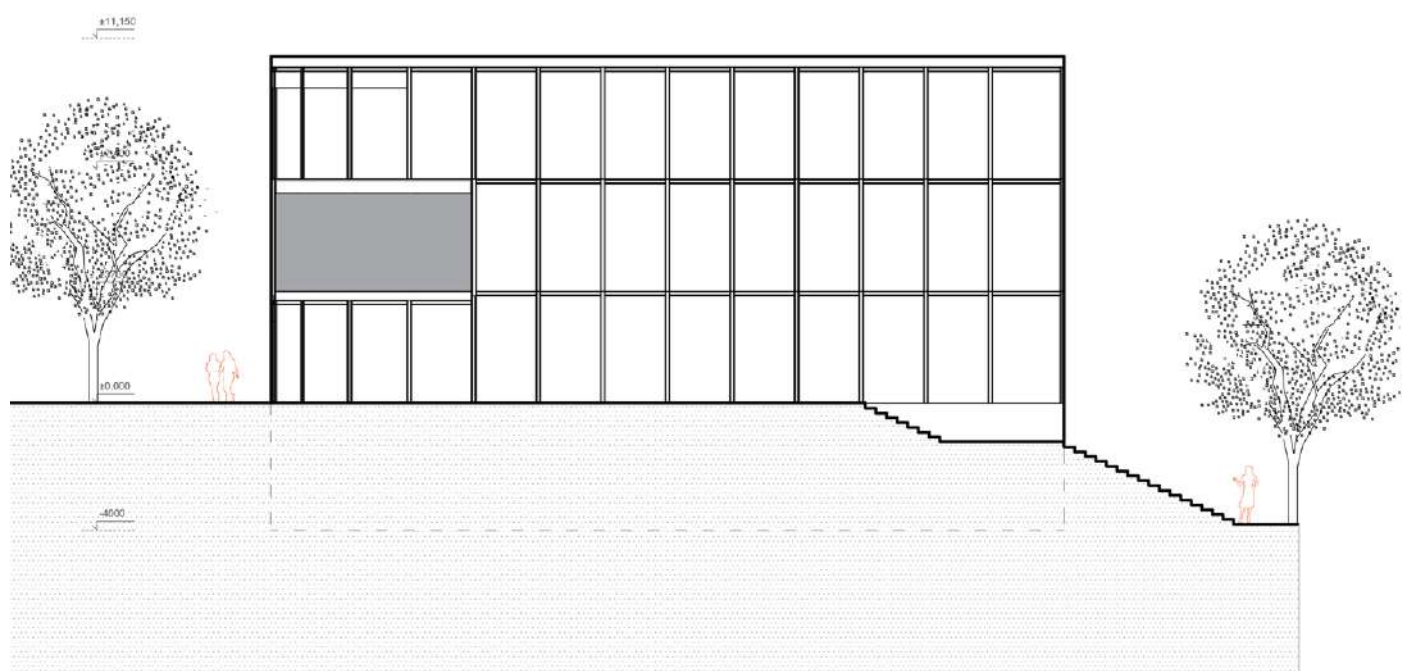
Pohľad severovýchodný M 1:250
