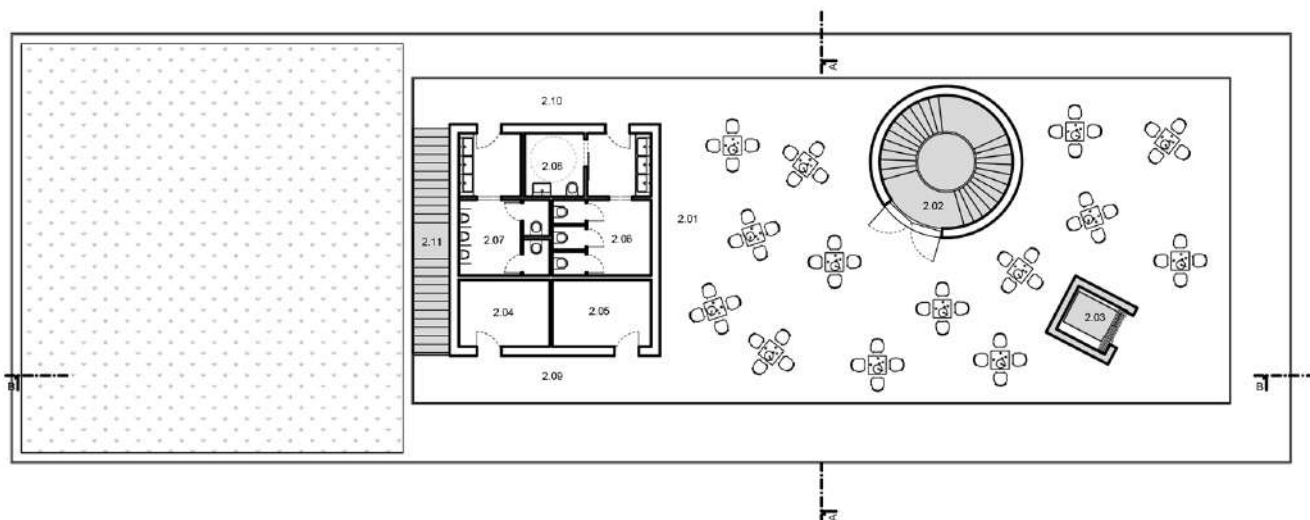
Pôdorys 2.NP M 1:250
