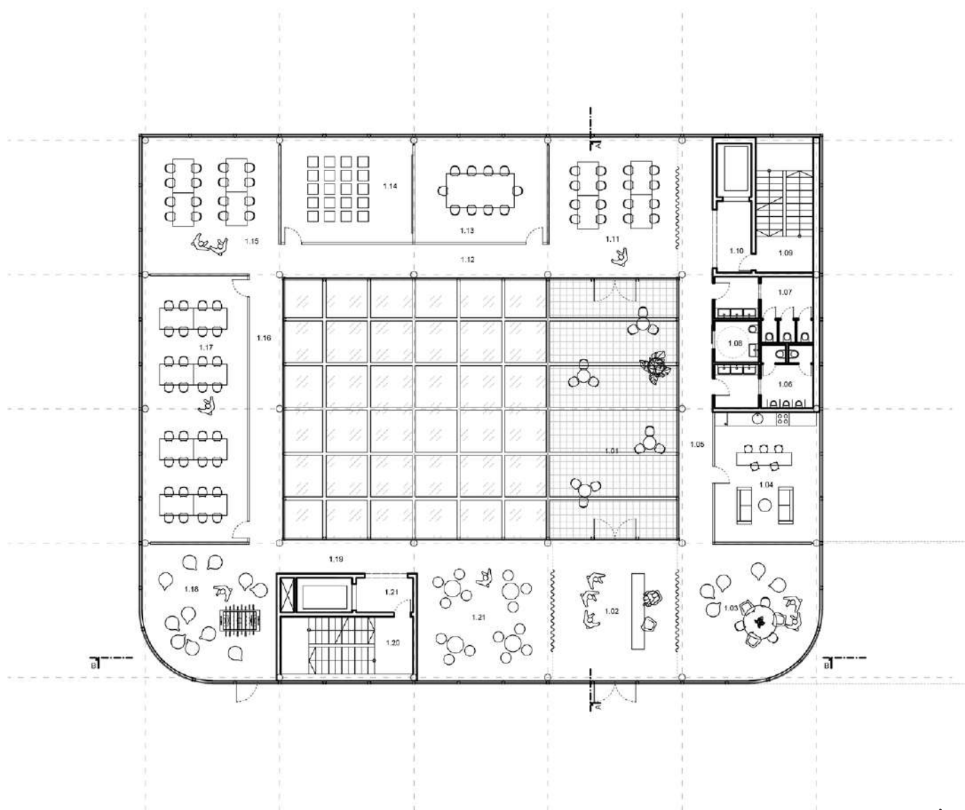
Pôdorys 1.NP M 1:250
