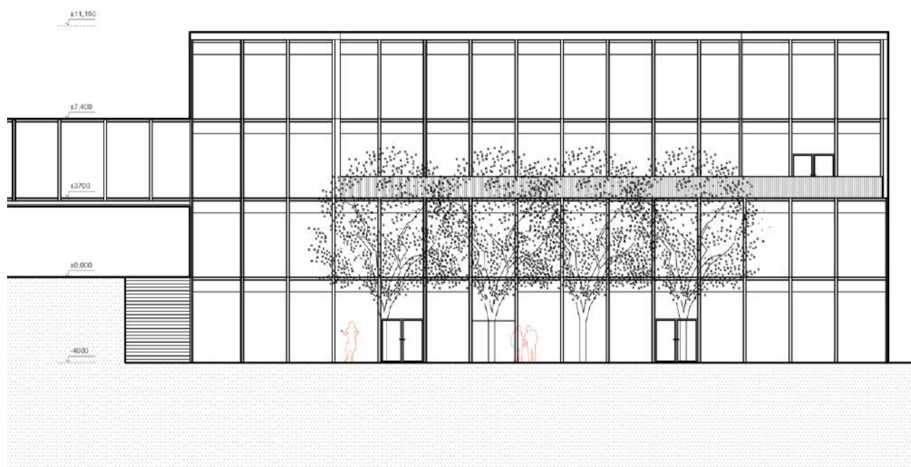
Pohľad severozápadný M 1:250
