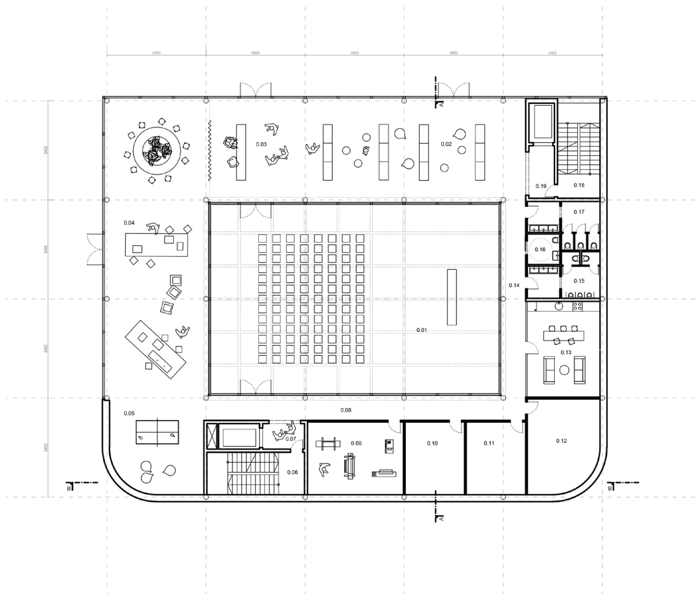
Pôdorys 1.PP M 1:250
