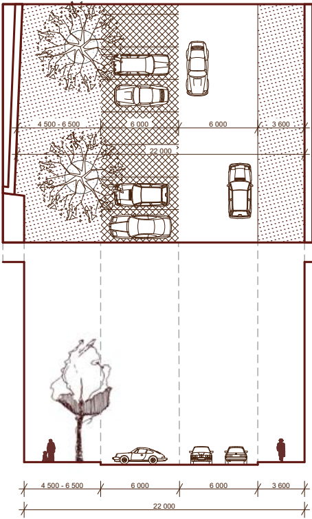
Navrhovaný stav
