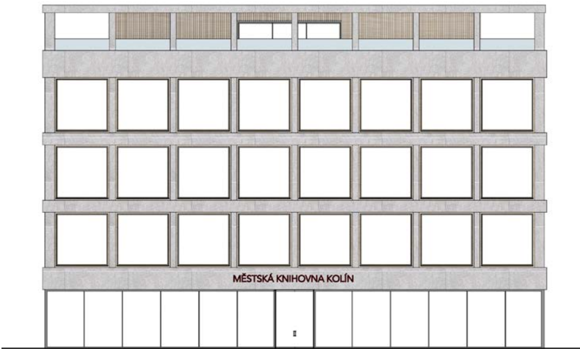
Pohled východní
