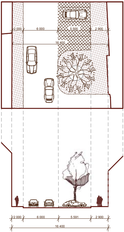
Navrhovaný stav
