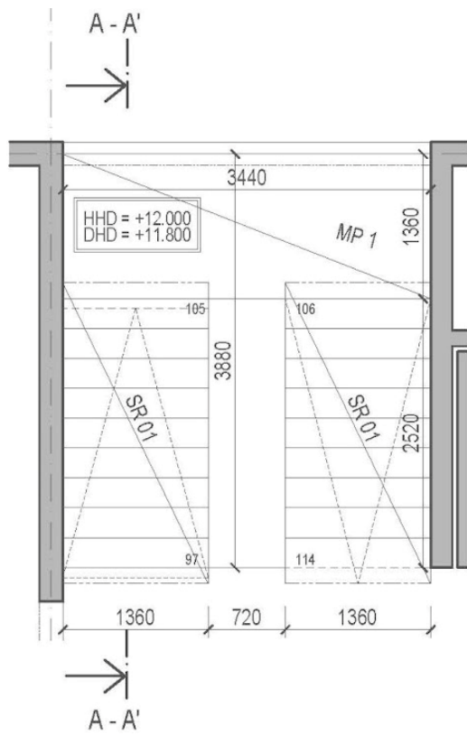
Obrázek D.2.2 - Půdorys schodiště
