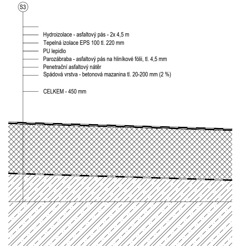
SKLADBA PODLAHY STŘECHA NEPOCHOZÍ NA NÁSTAVBĚ
