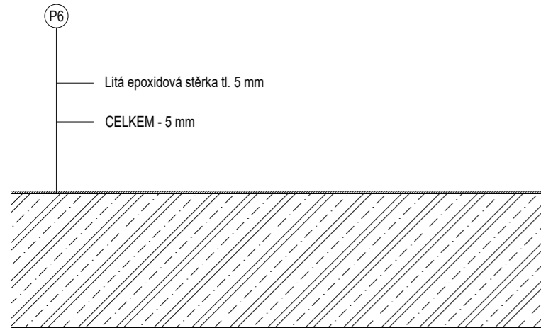
SKLADBA PODLAHY GARÁŽE A PROSTORY V 1PP
