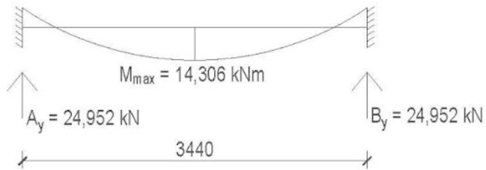
Obrázek D.2.5 - Schéma průběhu momentu na mezipodestě
