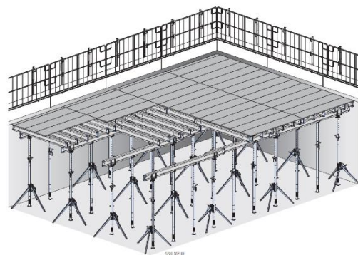
Obrázek č 4: Vodorovné bednicí prvky [3]
