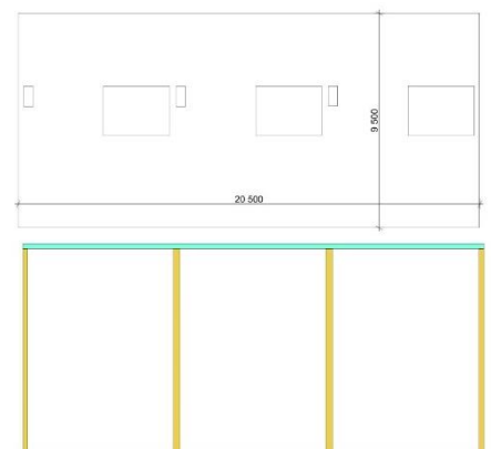
Obrázek č 2: Stropní deska a 2 záběry při betonáži zdí
