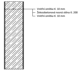
S2 SKLADBA VNITŘNÍ NOSNÉ STĚNY
