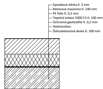
P1 SKLADBA PODLAHY- CHODBA + MÍSTNOSTI
