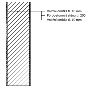
S3 SKLADBA NENOSNÉ DĚLÍČÍ PŘÍČKY
