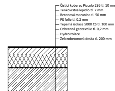
P5 SKLADBA PODLAHY- VSTUPNÍ MÍSTNOST
