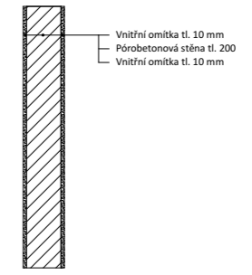
S4 SKLADBA NENOSNÉ DĚLÍČÍ PŘÍČKY
