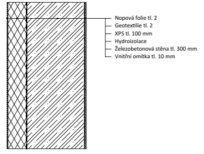
S5 SKLADBA OBVODOVÉ NOSNÉ STĚNY - ZAPUŠTĚNÉ
