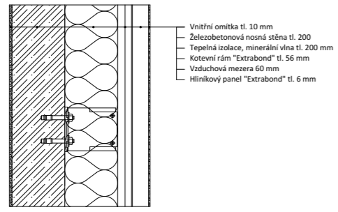
S5 SKLADBA OBVODOVÉ NOSNÉ STĚNY - ZAPUŠTĚNÉ
