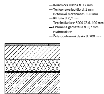
P4 SKLADBA PODLAHY- BAZÉN
