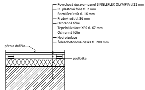
P6 SKLADBA PODLAHY- SPORTOVNÍ HALA
