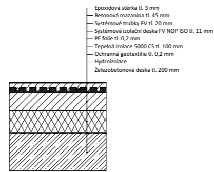
P2 SKLADBA PODLAHY- KMENOVÁ TŘÍDA
