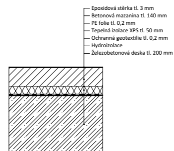
P8 SKLADBA PODLAHY- TECHNICKÁ MÍSTNOST
