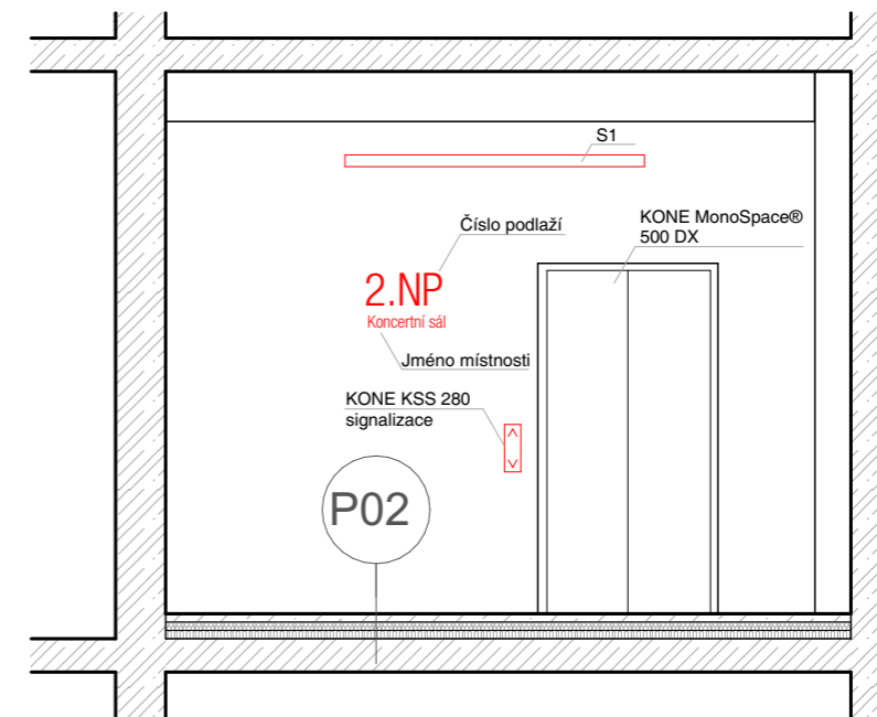
Řez A-A' 1:50
