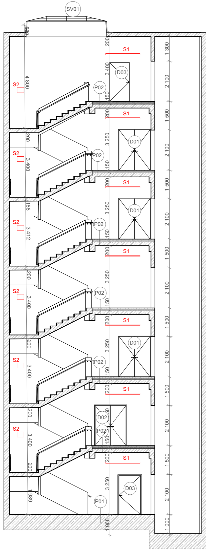
Řez B-B'
