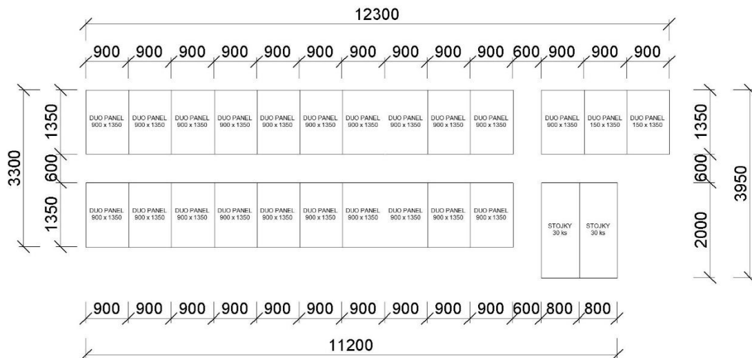
obr.č.7: schéma skladovania debnenia a stojok
