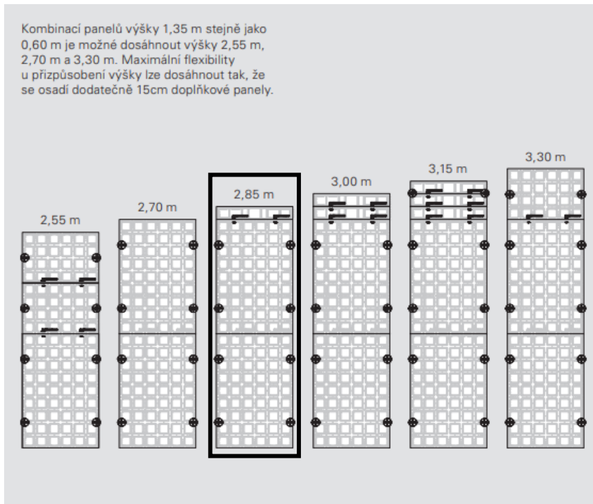
obr.č.6: kombinácia prefabrikátov debnenia PERI DUO
